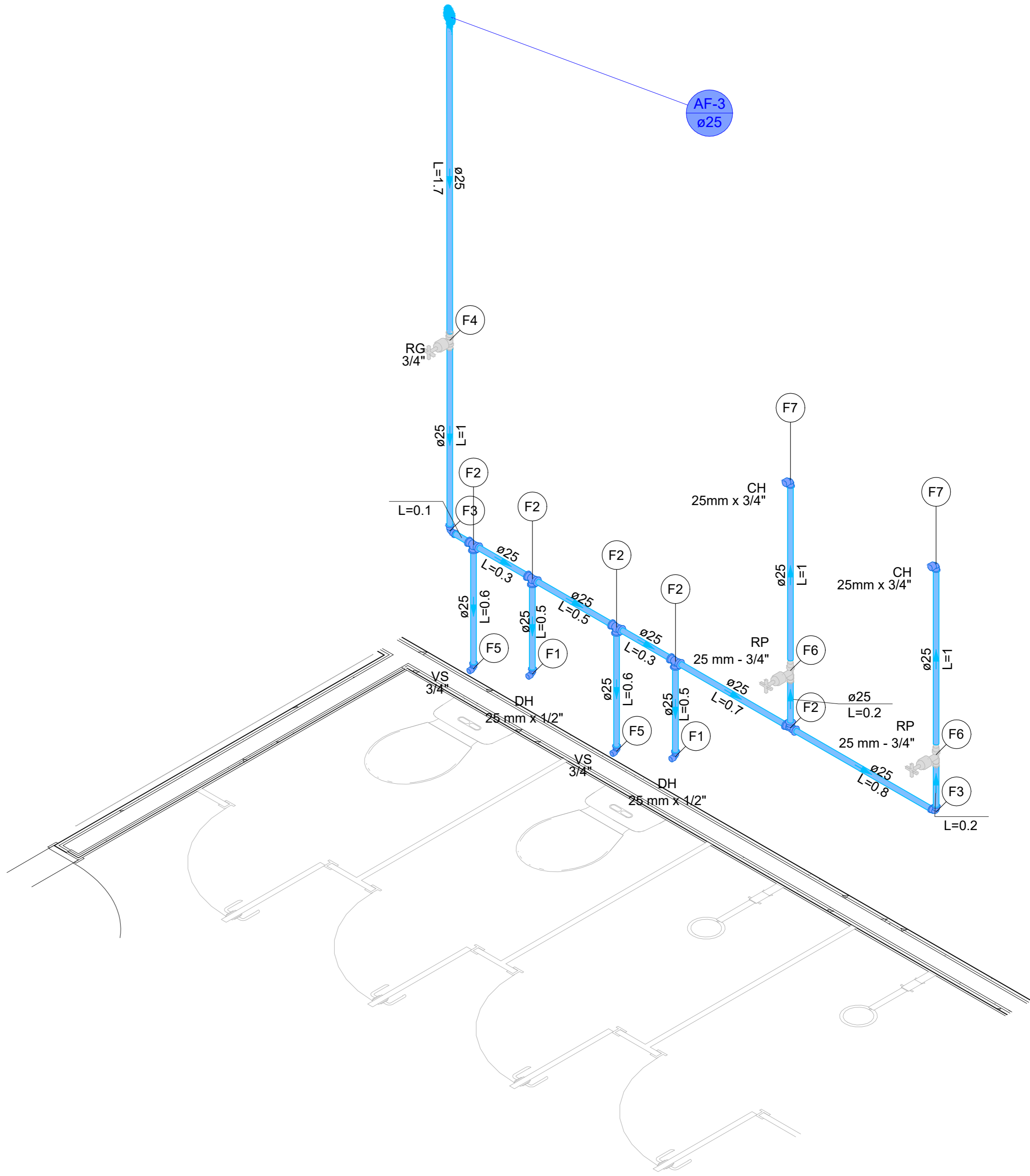
DETALHE HID-2 1:25
