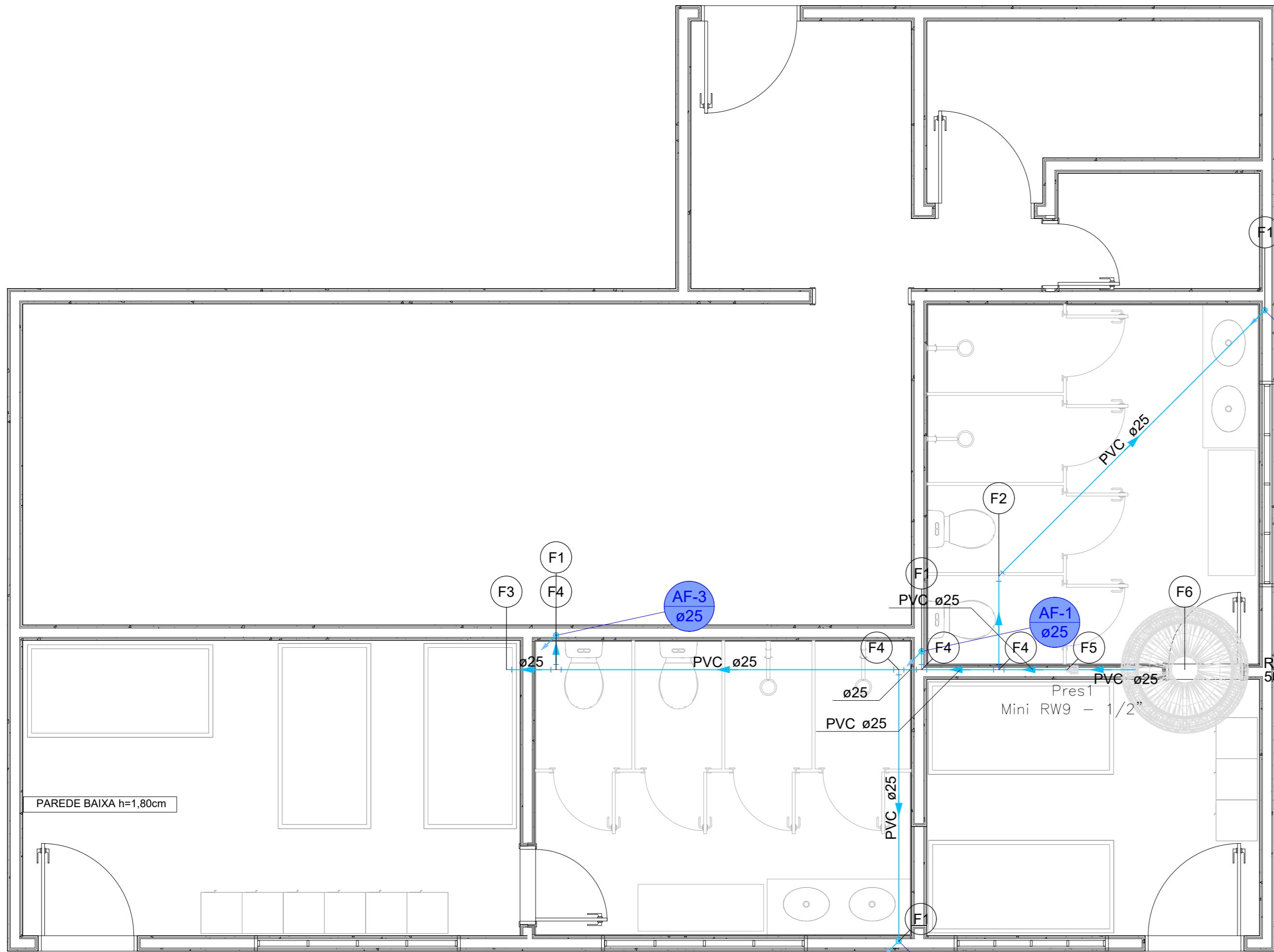
PLANTA DE COBERTURA-HIDRAULICO ESC. 1/50
