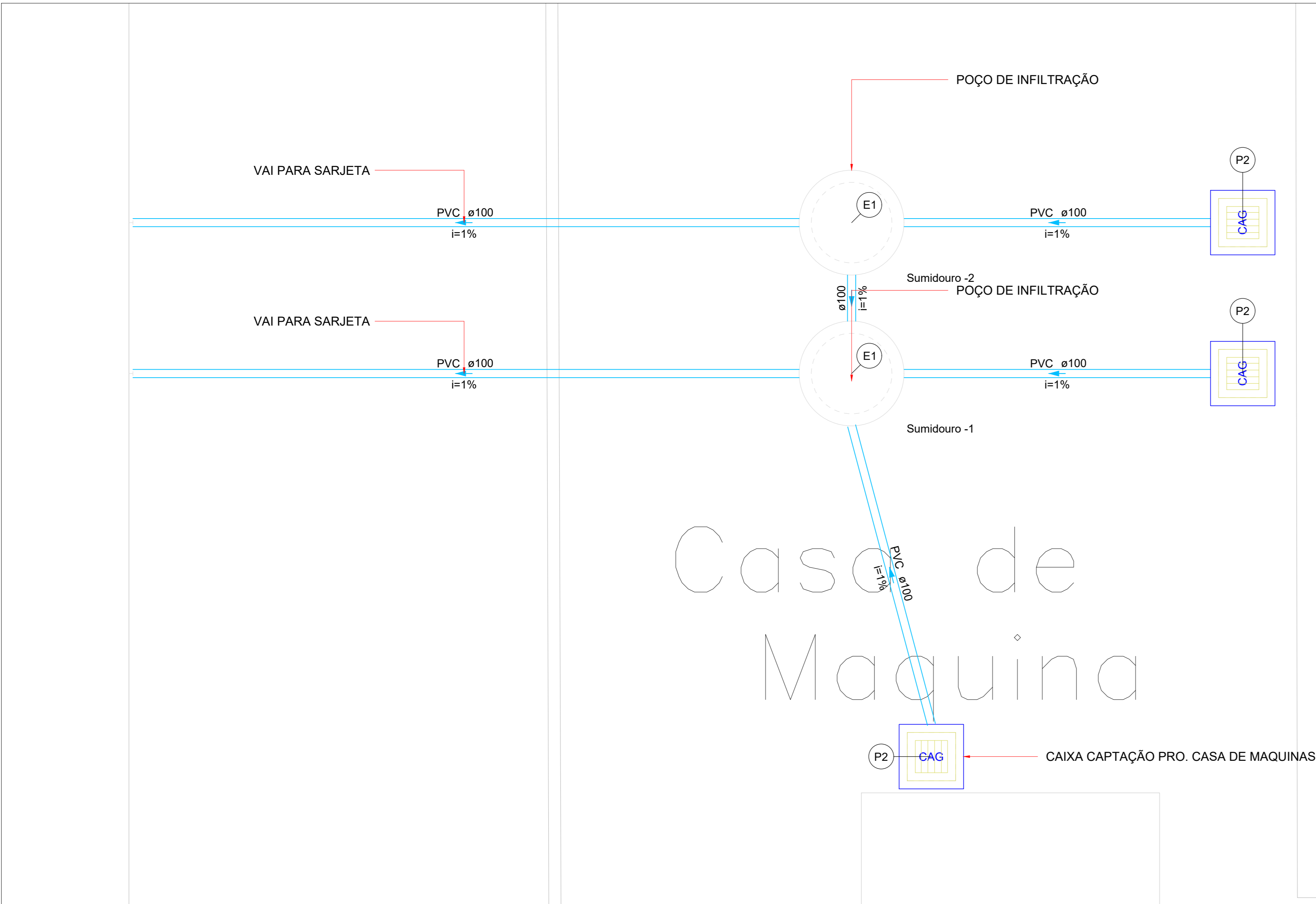
PLANTA DE BAIXA - DRENAGEM PISCINA ESC. 1/50
