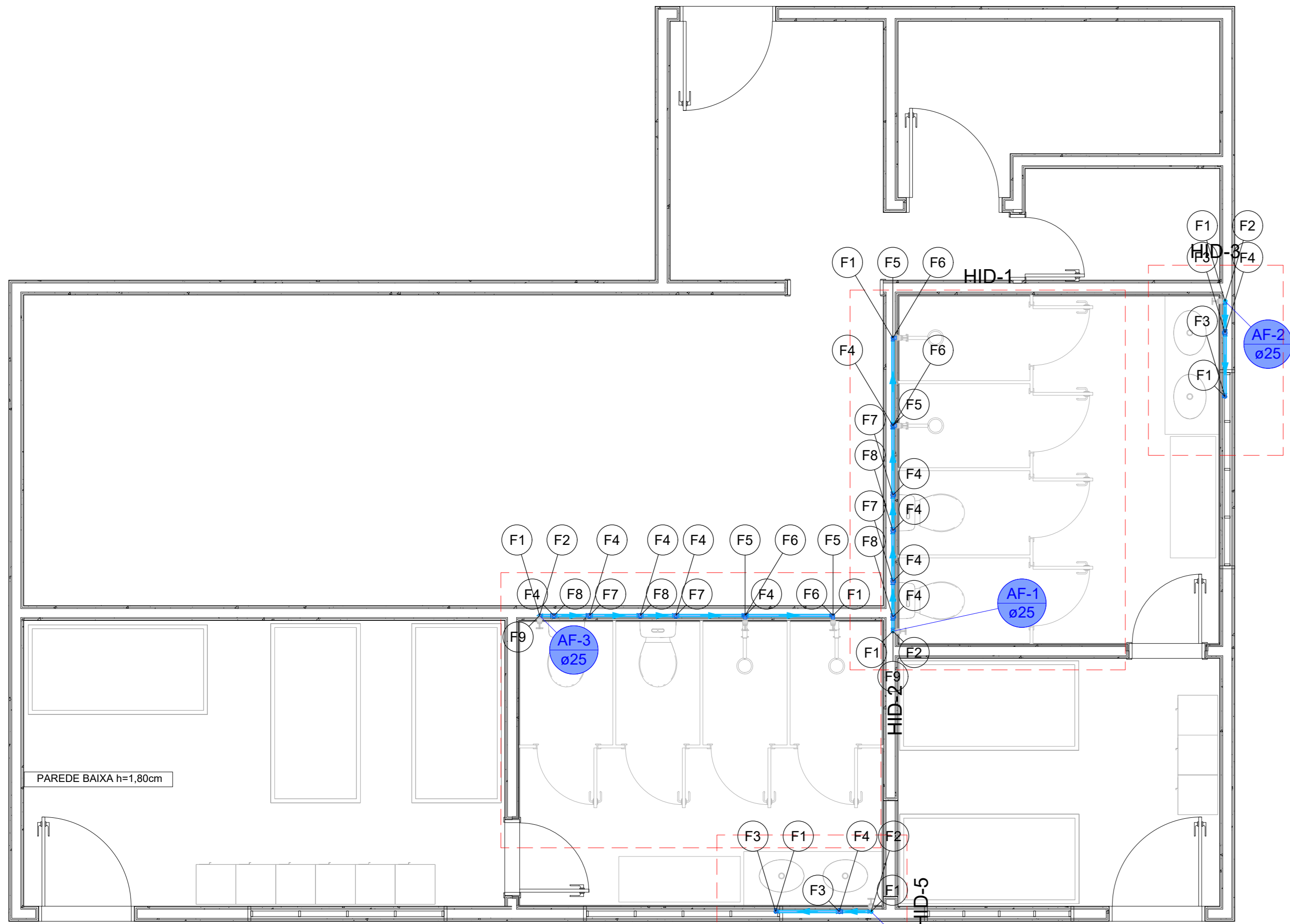
PLANTA DO TÉRREO - HIDRAULICO ESC. 1/50
