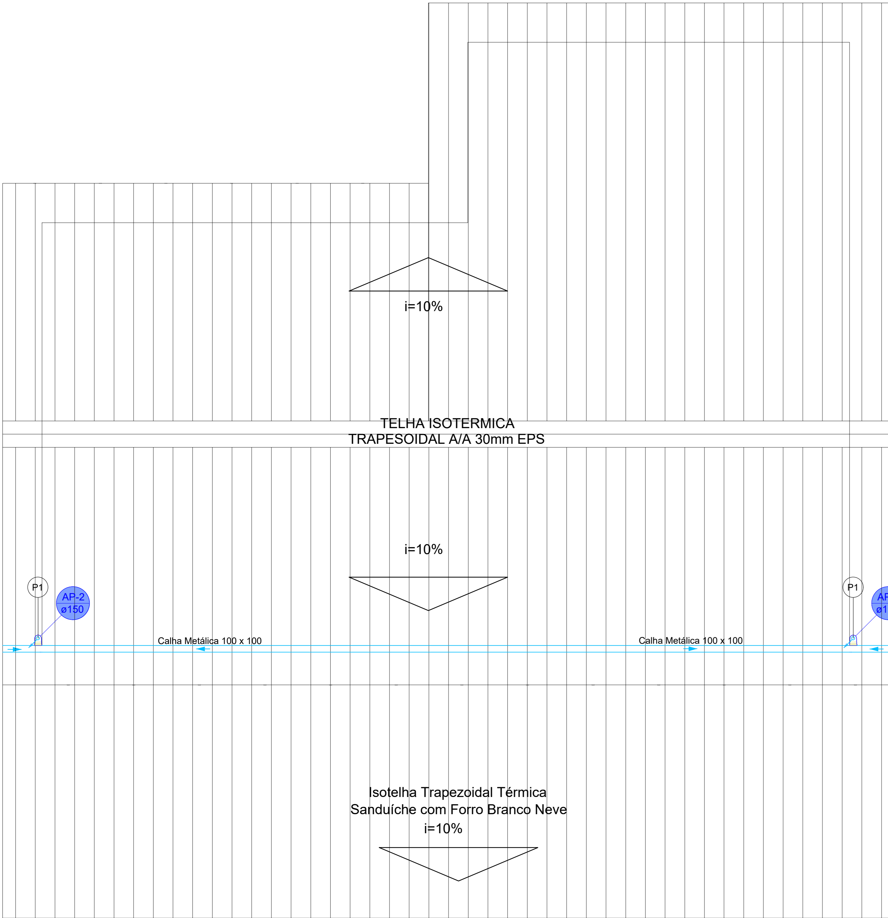
PLANTA DE COBERTURA - PLUVIAL ESC. 1/50
