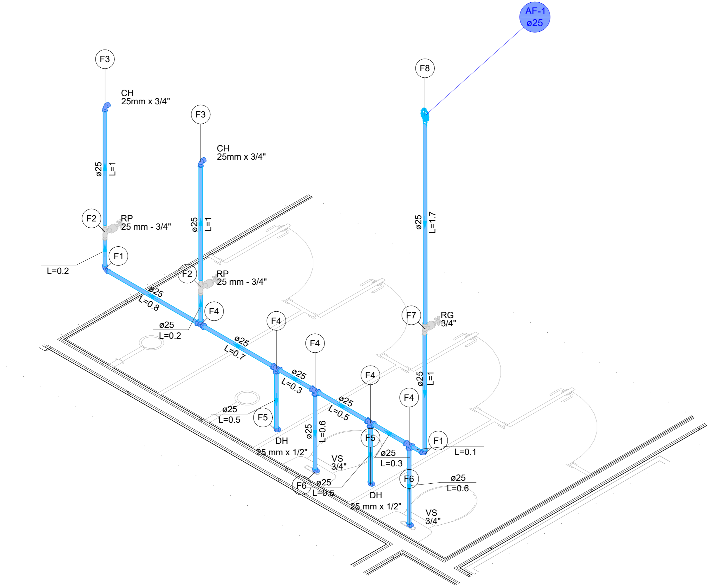
DETALHE HID-1 1:25
