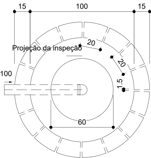
POÇO - TÉRREO Planta baixa - ESC. 1:25
