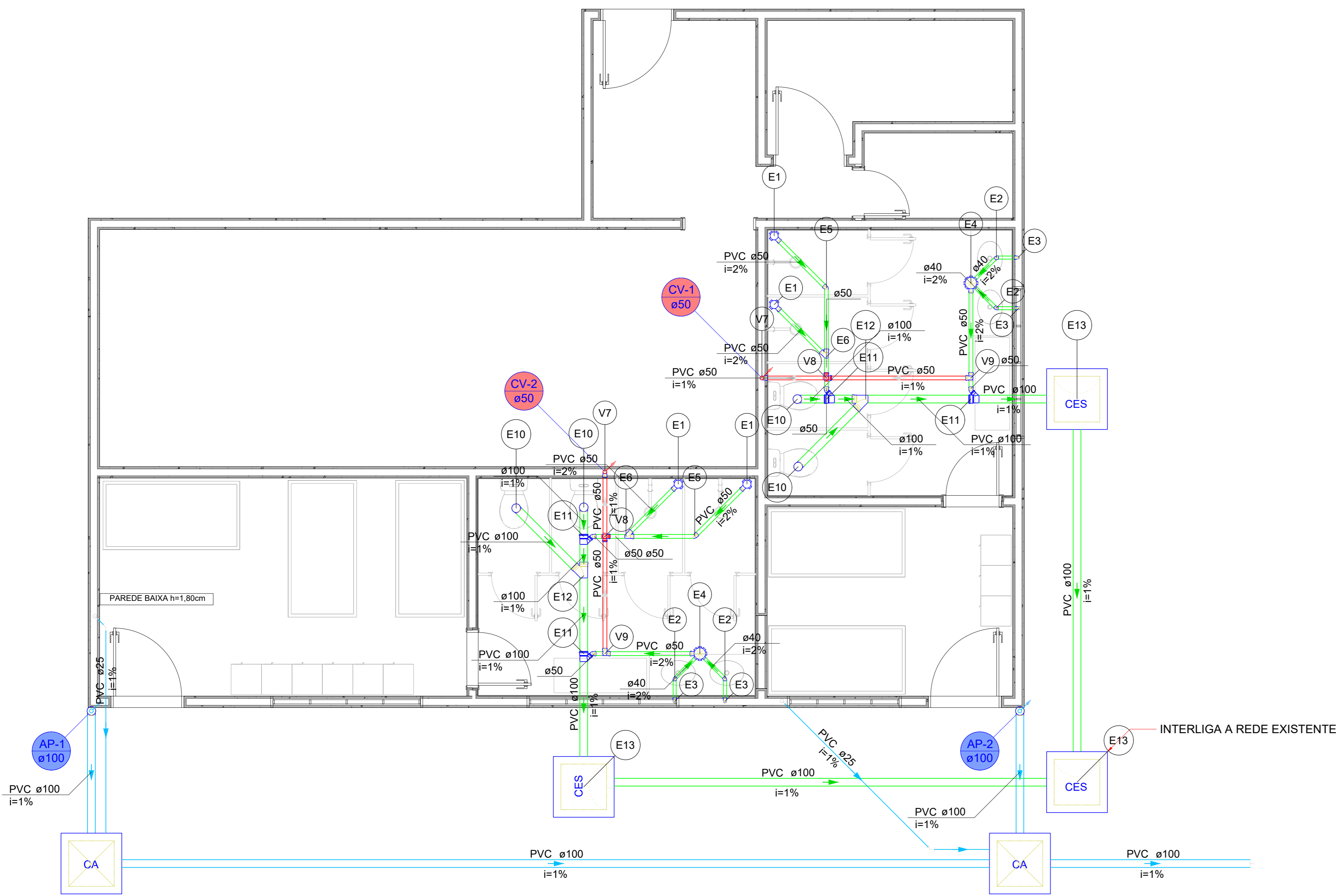
PLANTA DO TERREO - SANITÁRIO ESC. 1/50
