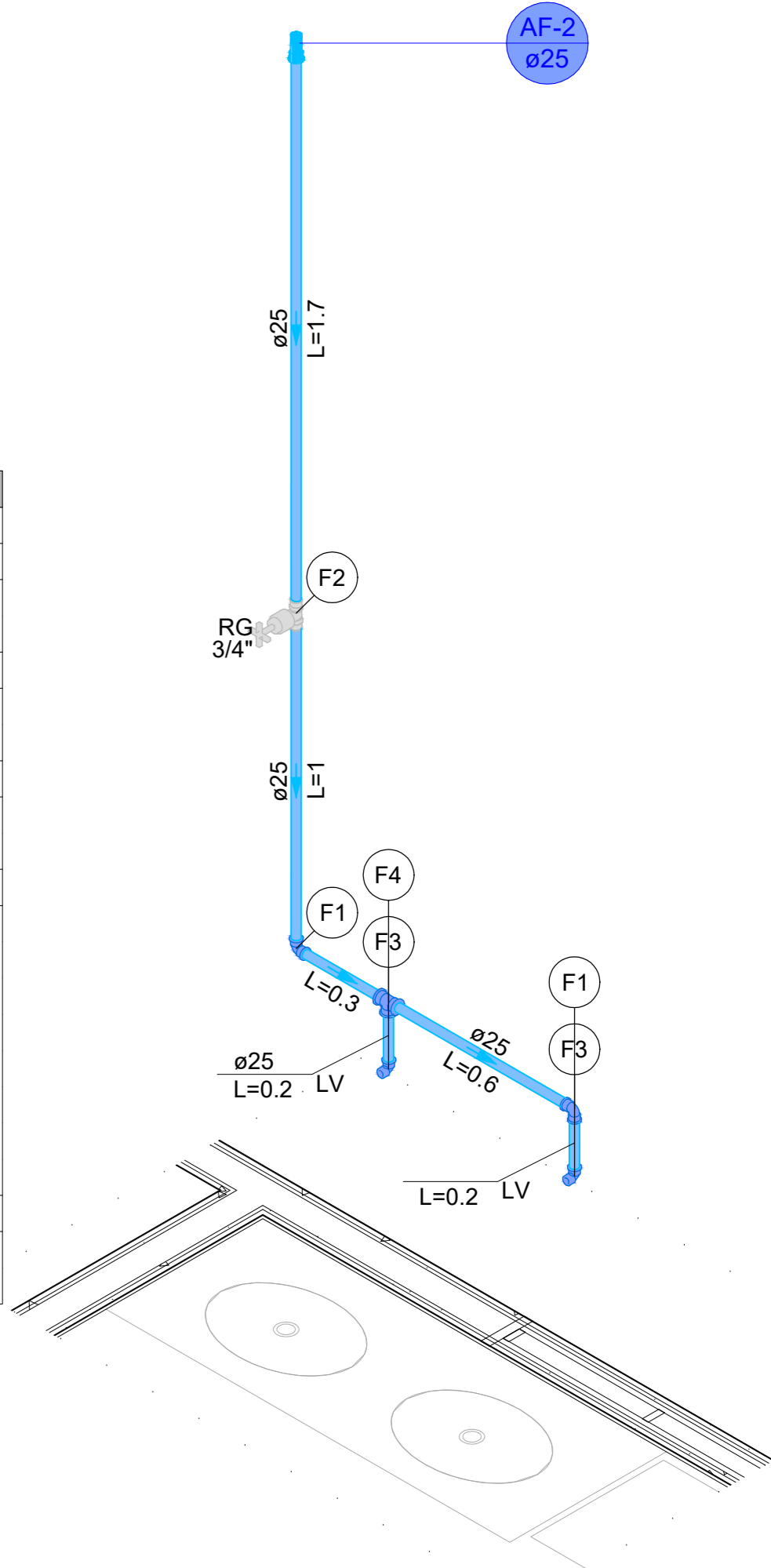
DETALHE HID-3 1:25
