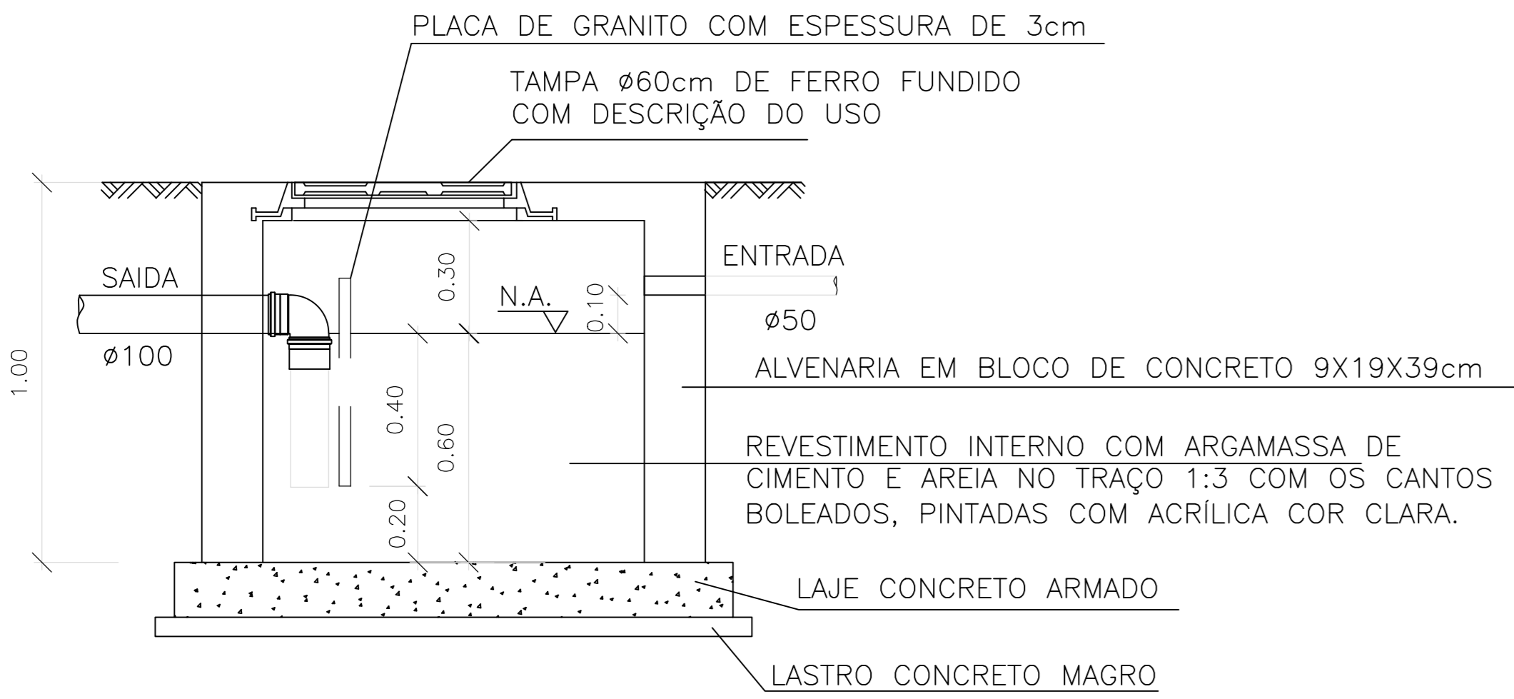
CORTE AA – CAIXA DE GORDURA ESPECIAL (CGE)
