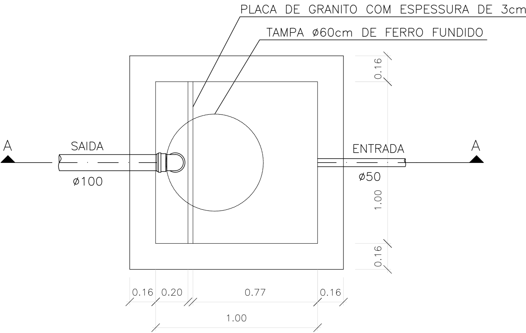
PLANTA BAIXA – CAIXA DE GORDURA ESPECIAL (CGE)
