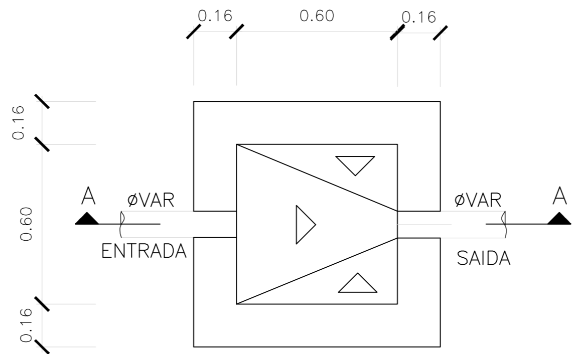
PLANTA BAIXA – CAIXA DE INSPEÇÃO (CI)
