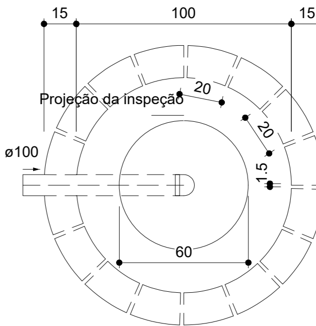
POÇO - TÉRREO Planta baixa - ESC. 1:25
