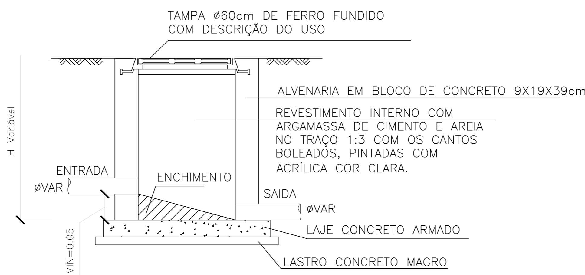
CORTE AA – CAIXA DE INSPEÇÃO (CI)
