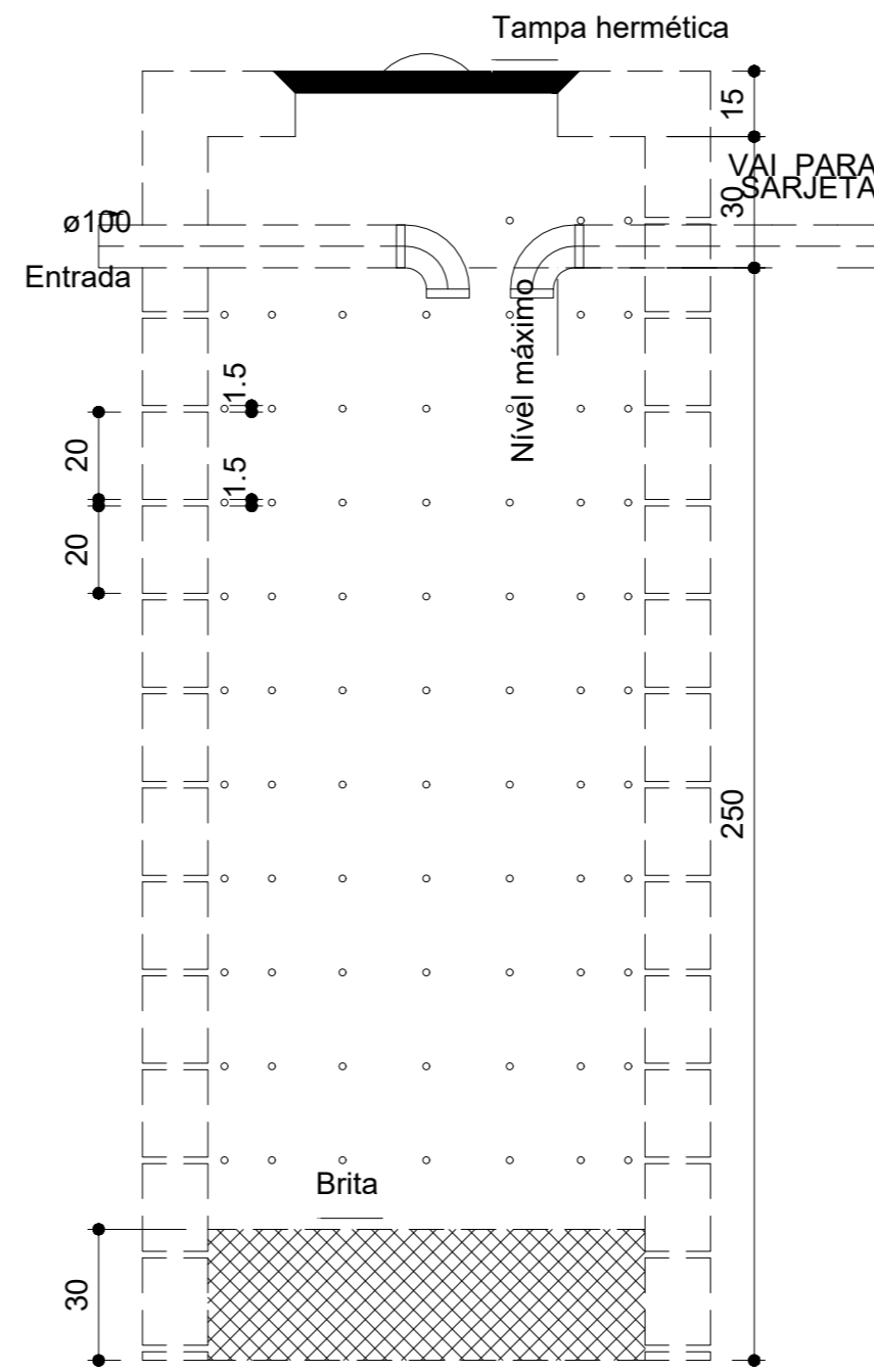
POÇO - TÉRREO Corte 1 - ESC. 1:25
