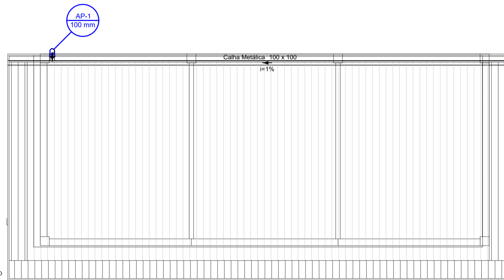
PLANTA DE COBERTURA SANITÁRIO ESCALA 1/50
