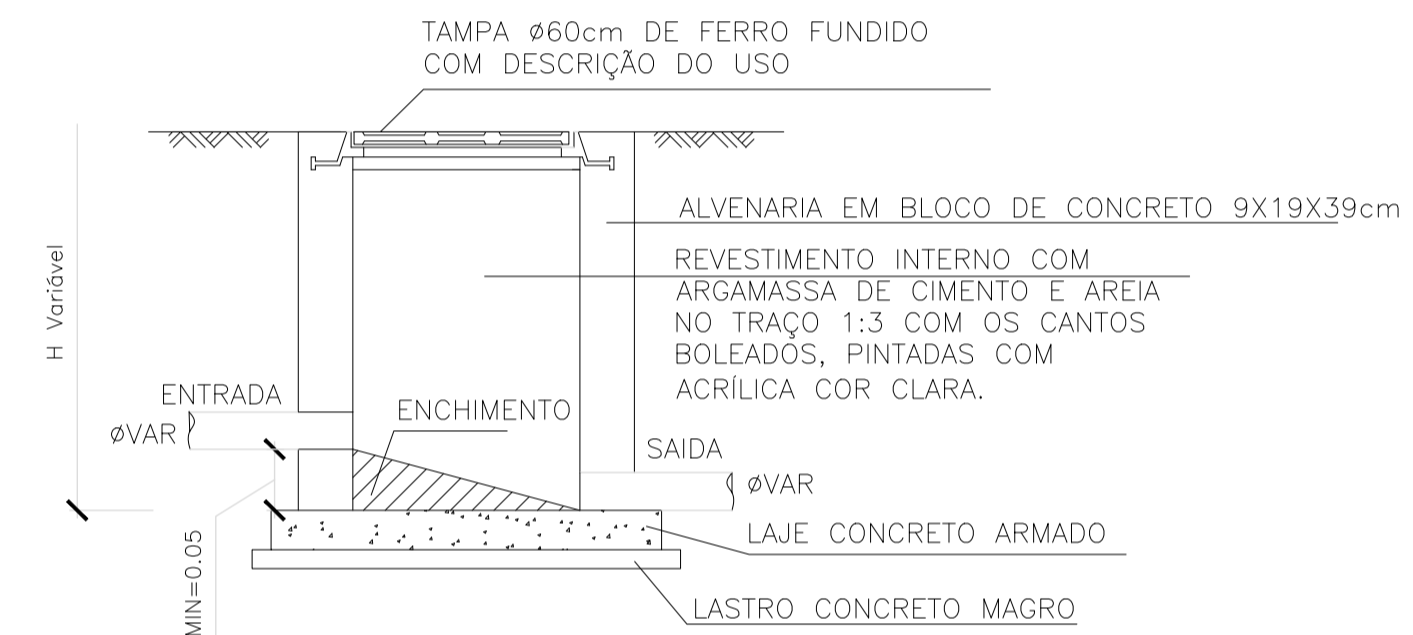
CORTE AA - CAIXA DE INSPEÇÃO (CI) ESCALA 1:25
