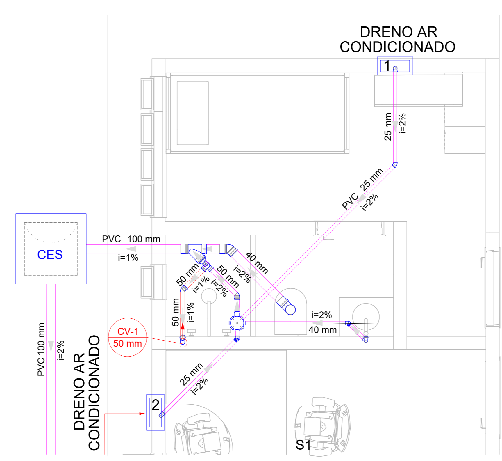
Detalhe S1 Escala 1:25
