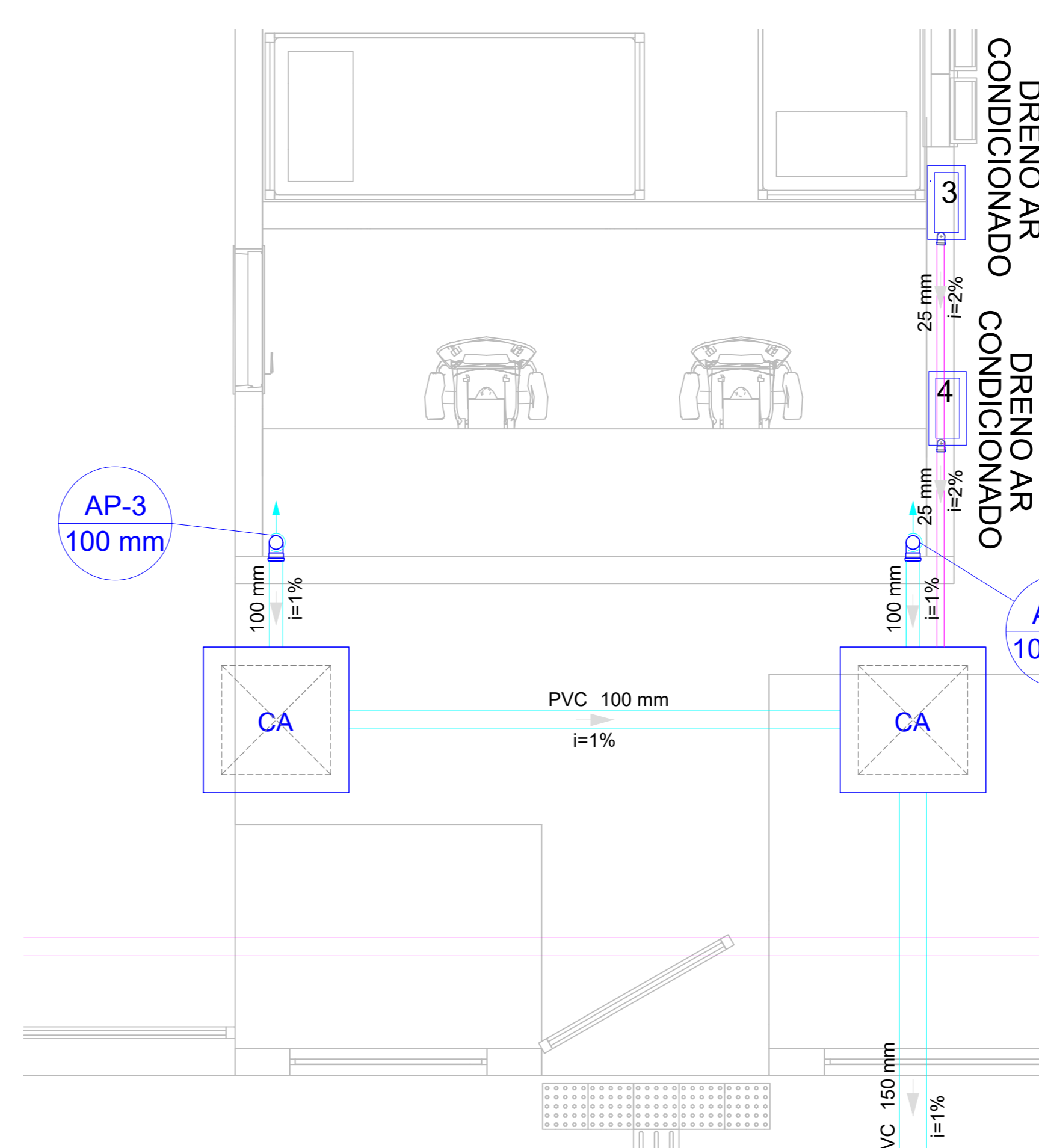
Detalhe S1 Escala 1:25
