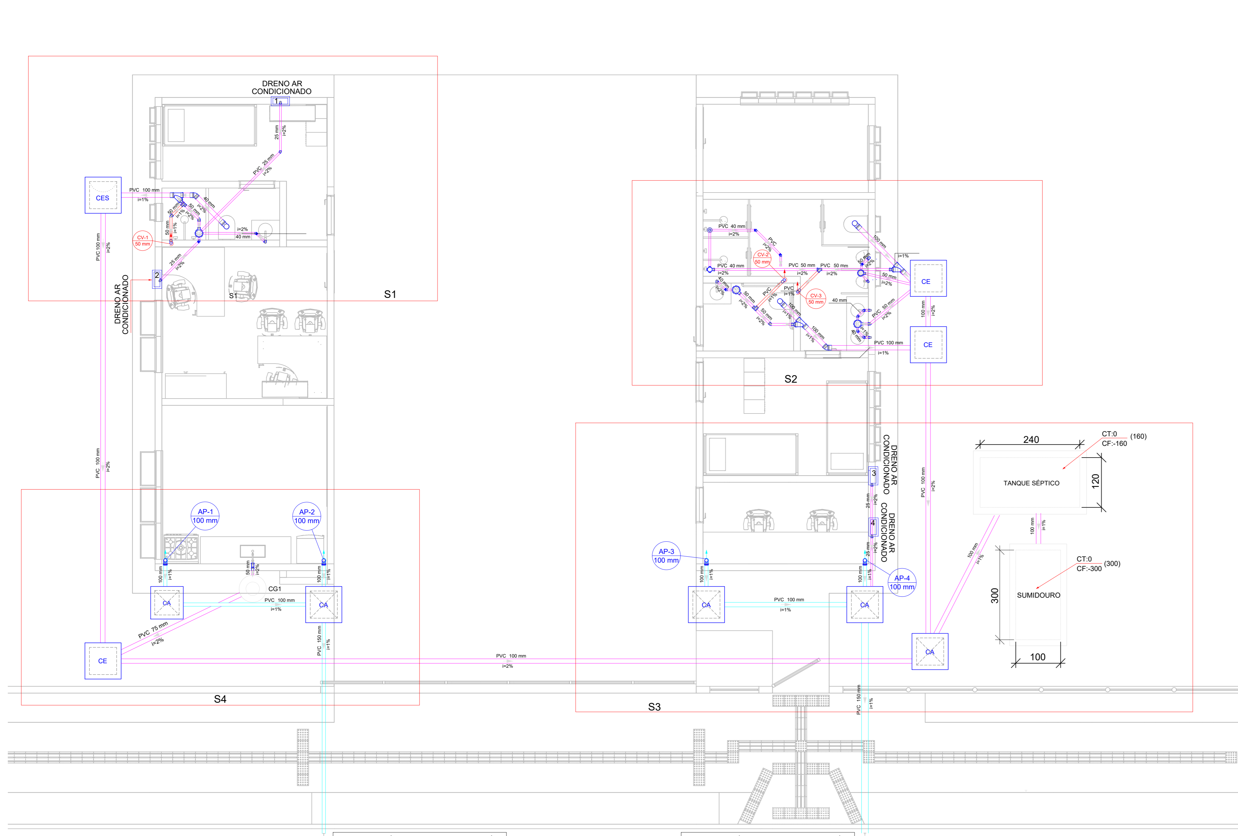
Planta Baixa Térreo Escala 1:50
