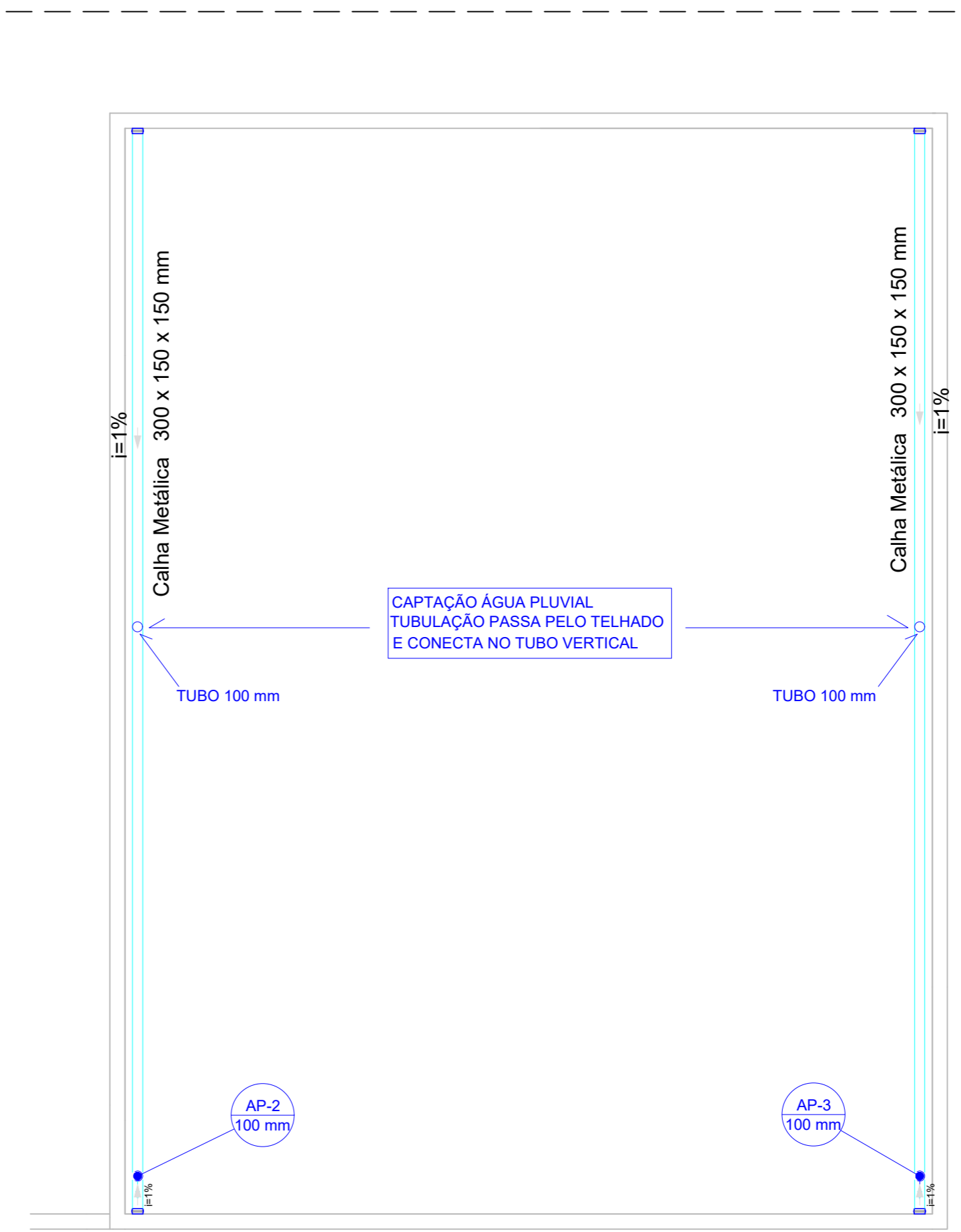
Planta Cobertura Garagem Operacional Escala 1:50
