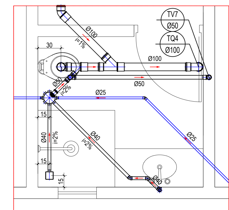
Detalhe S5 Escala 1:25
