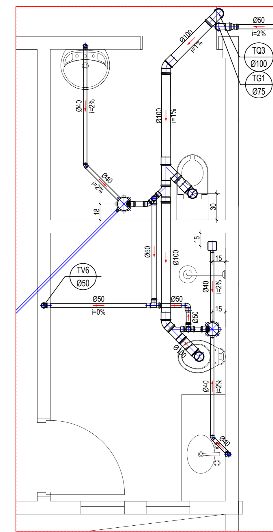
Detalhe S3 Escala 1:25
