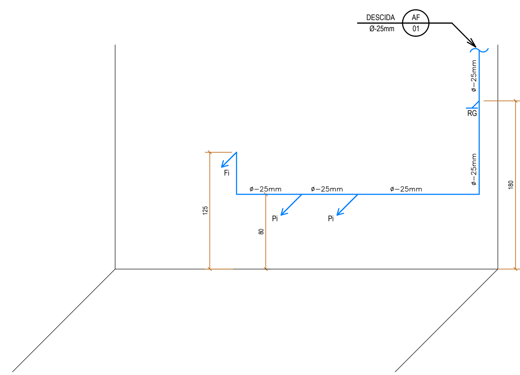
ISOMÉTRICA A Escala 1/25
