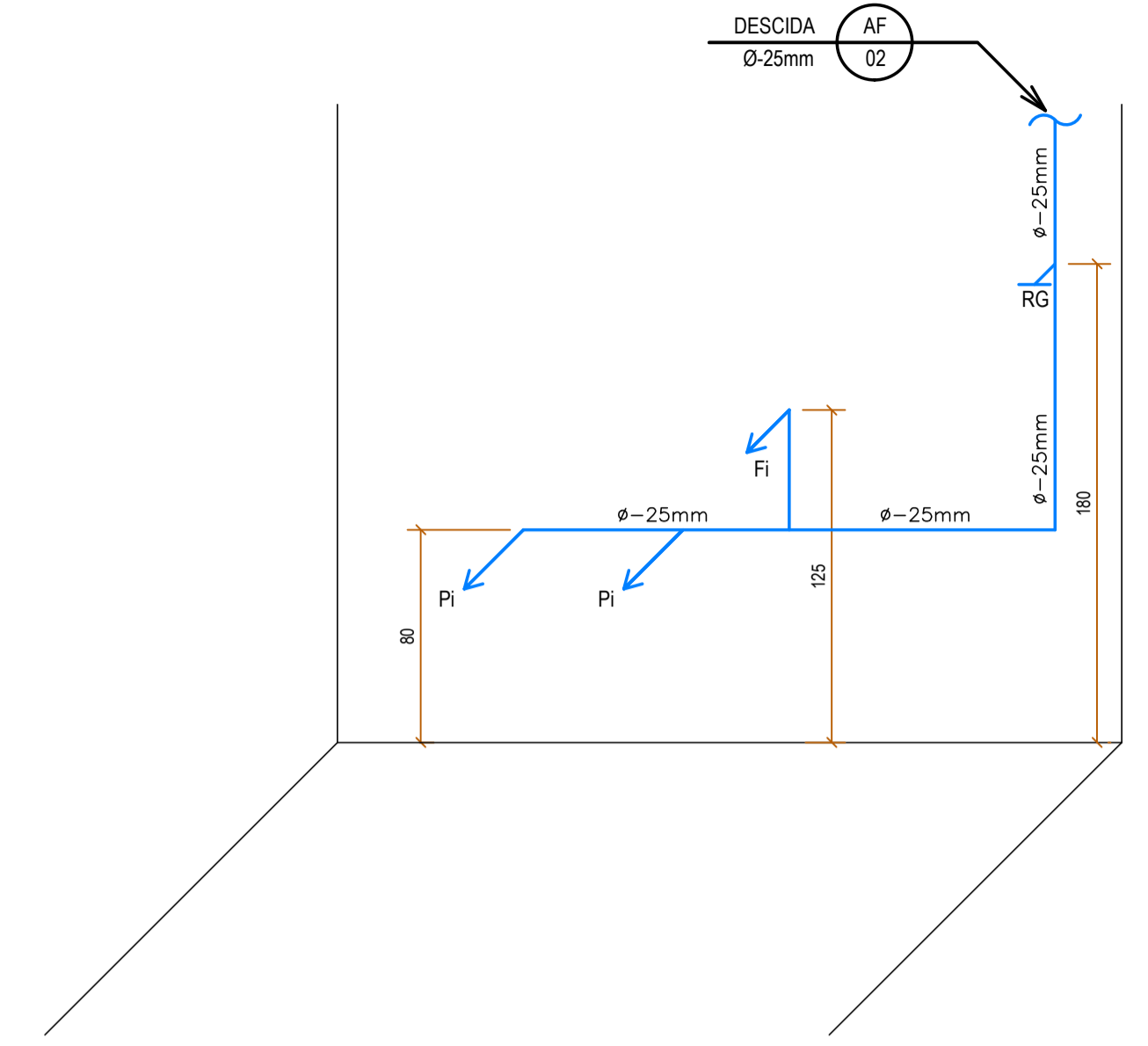
ISOMÉTRICA B Escala 1/25
