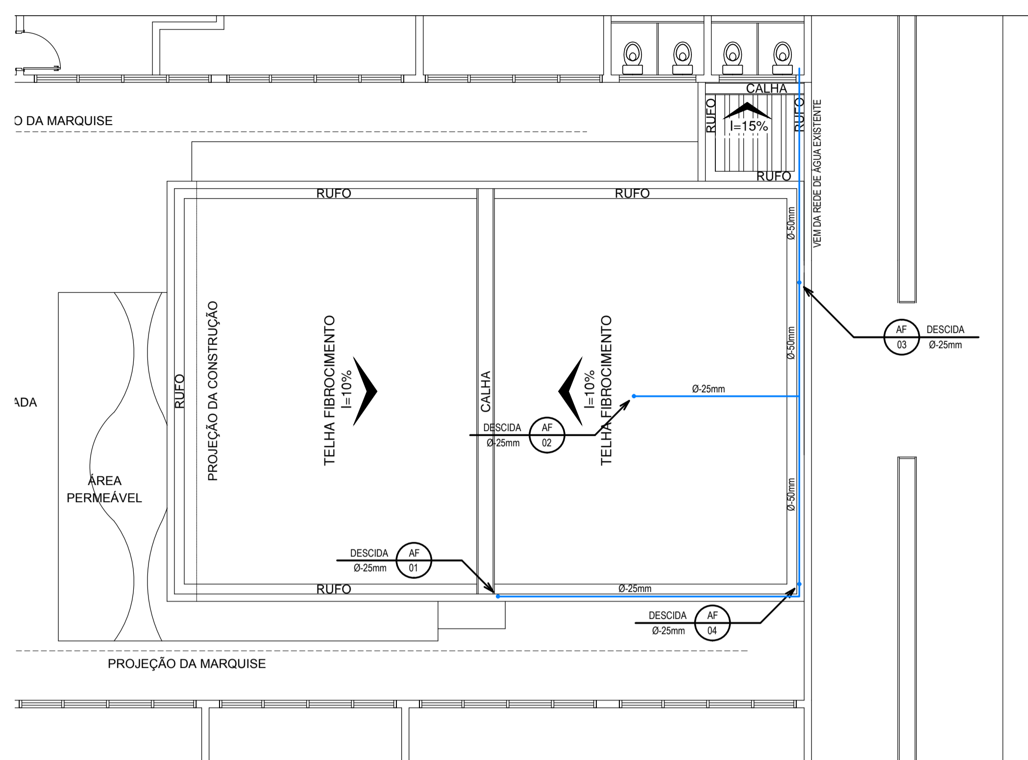
PLANTA DE COBERTURA - MODIFICAÇÃO - REFEITÓRIO E COPA ESC.: 1/75 Área Construída=109,14m2
