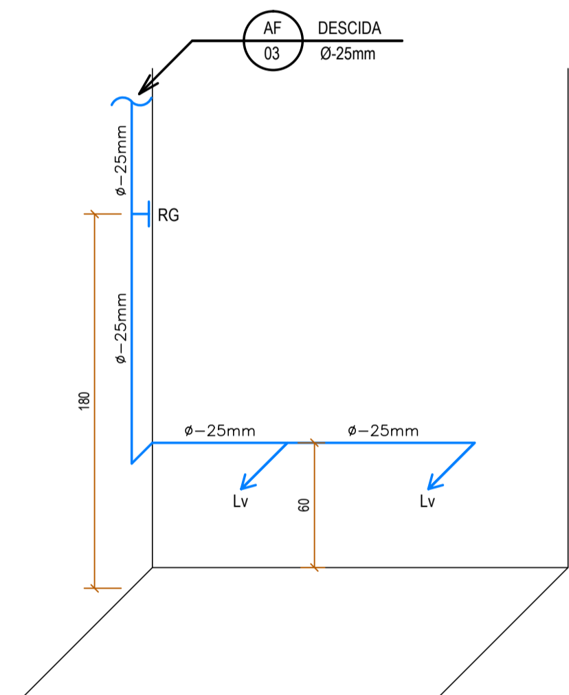
ISOMÉTRICA C Escala 1/25
