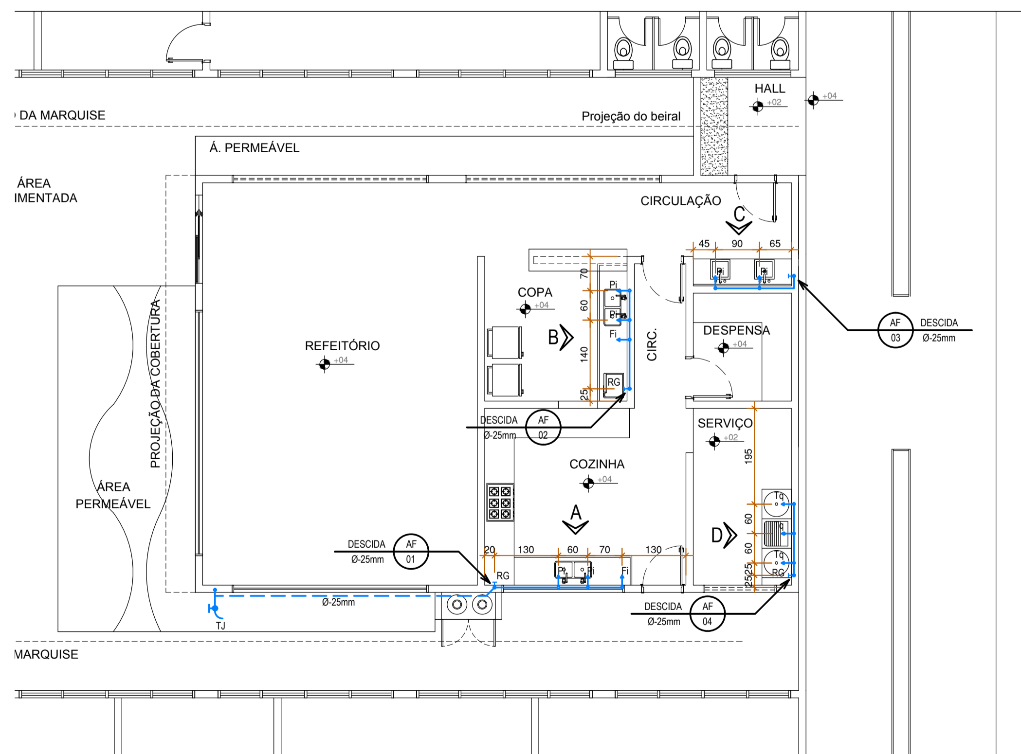
PLANTA BAIXA - MODIFICAÇÃO - REFEITÓRIO E COPA ESC.: 1/75 Área Construída=109,14m2
