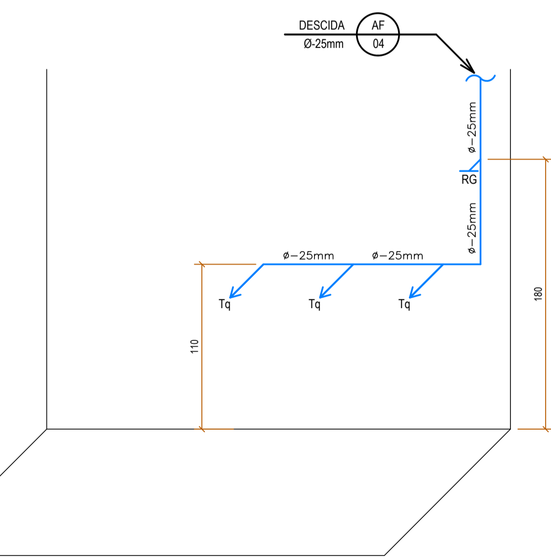
ISOMÉTRICA D Escala 1/25
