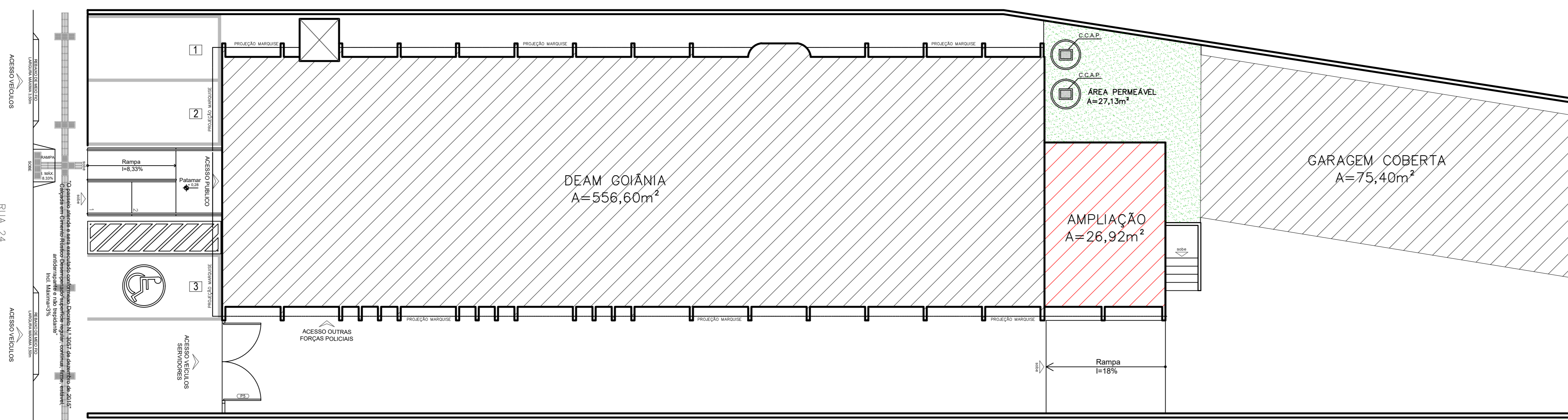
IMPLANTAÇÃO escala: 1/100
