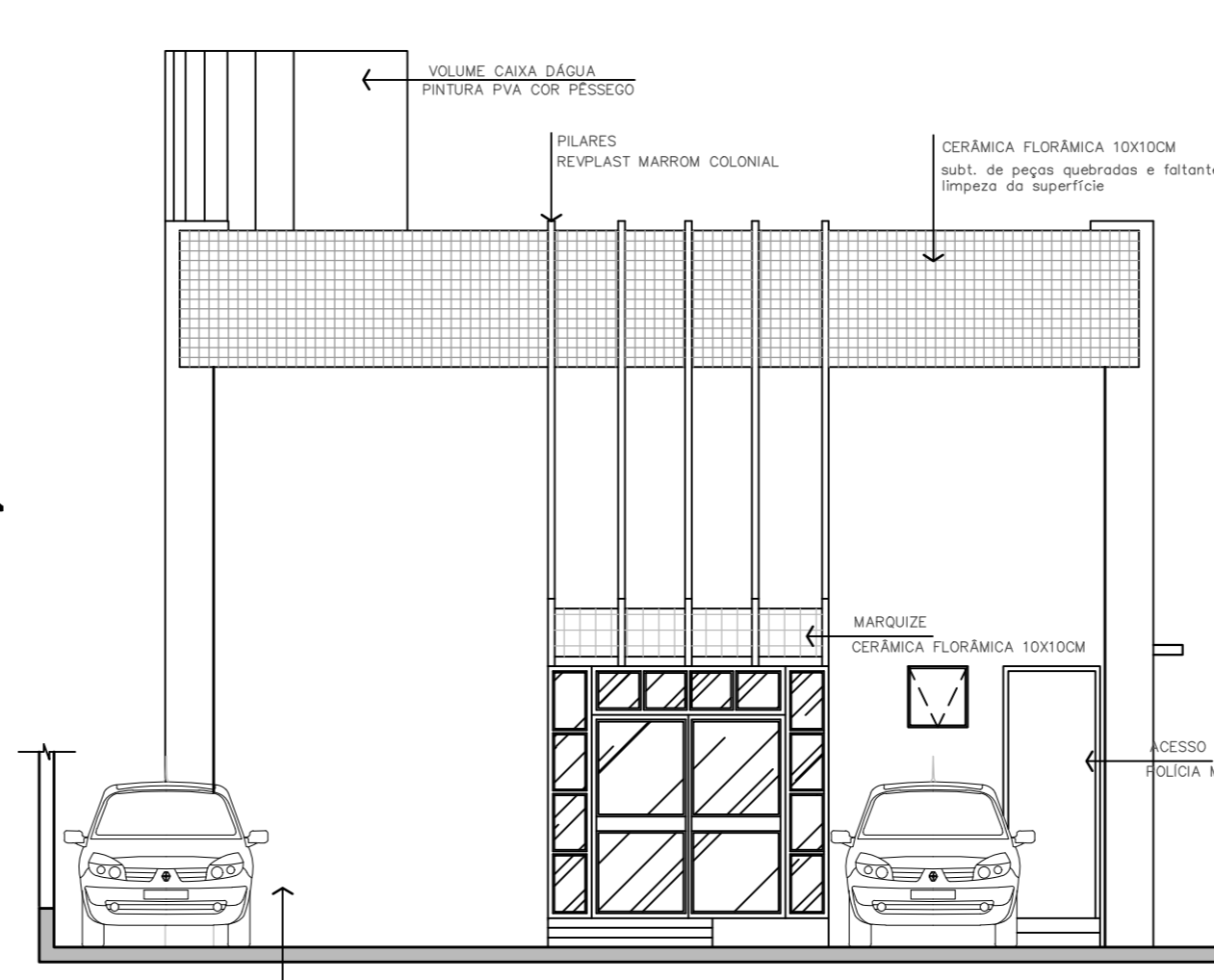
FACHADA FRONTAL escala: 1/75
