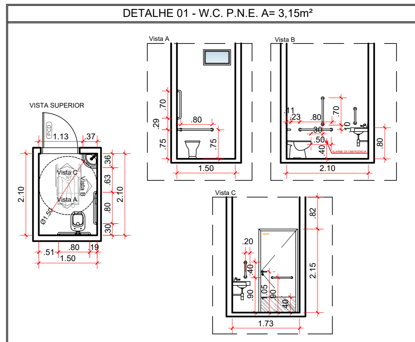
DET. WC P.N.E. escala: 1/50
