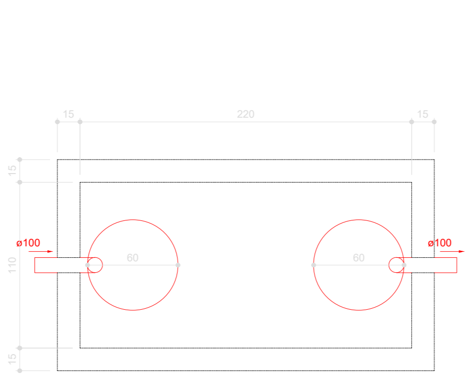
Tanque séptico Planta baixa - ESC. 1:25
