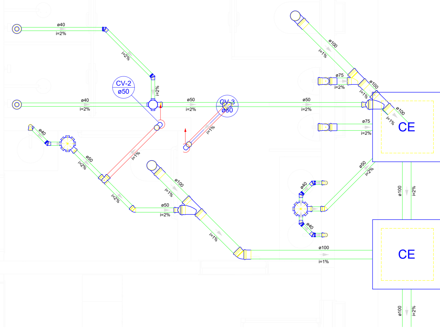
Detalhe S2 Escala 1:25
