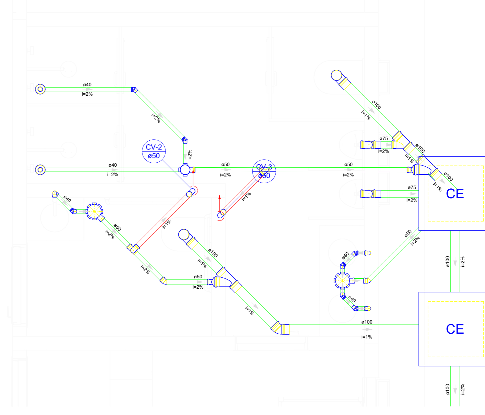
Detalhe S2 Escala 1:25
