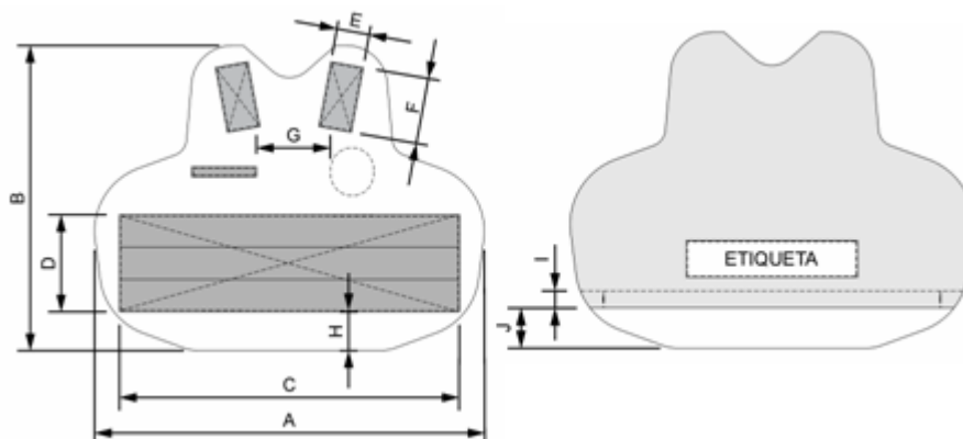
DIMENSÕES CAPA FRONTAL - MODELO MASCULINO (m.m.) TOLERÂNCIA: ± 5M.M (MAIS OU MENOS CINCO MILÍMETROS)
