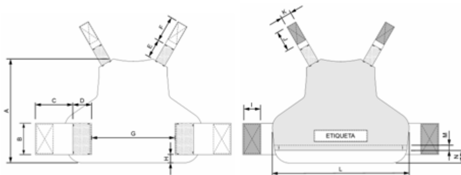
DIMENSÕES CAPA DORSAL – MODELO MASCULINO (mm) TOLERÂNCIA: ± 5M.M (MAIS OU MENOS CINCO MILÍMETROS)
