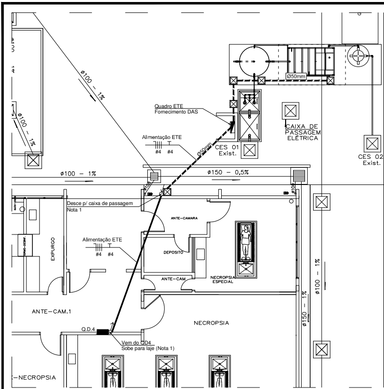
PLANTA BAIXA - TERREO ESCALA 1:10
