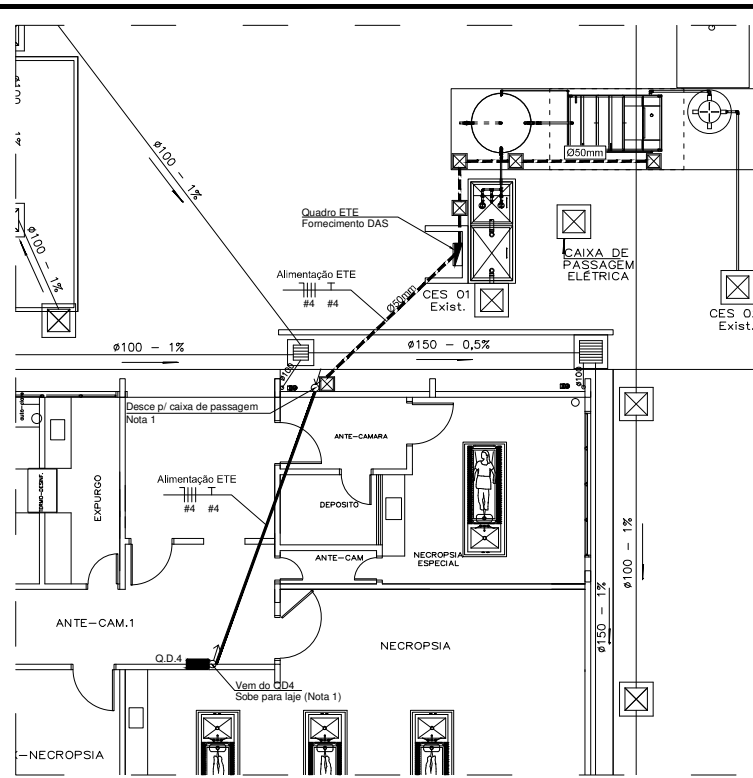
PLANTA BAIXA - TERREO ESCALA 1:10
