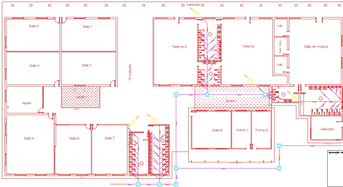
ESC. 1:100 PLANTA BAIXA – TÉRREO Salas de Aula – ADEQUAÇÃO / REFORMA
