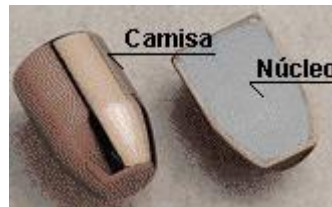
Imagem 01: Projétil ETPP.
