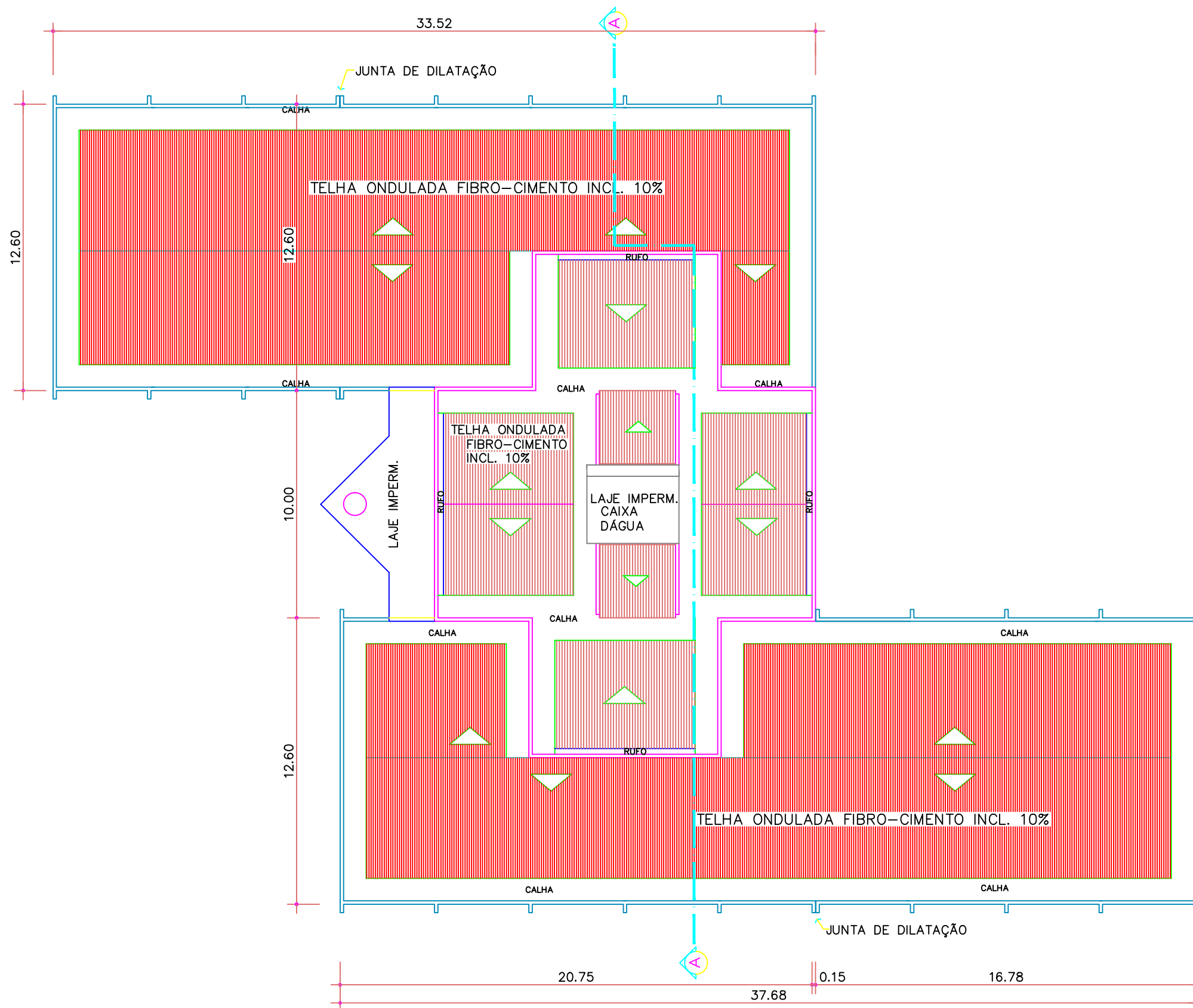
PLANTA DE COBERTURA ESC: 1/200
