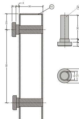
Fig. 10 – Sistema de encaixe Longarinas escala 1:1 (em mm)
