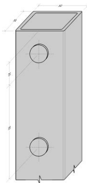
Fig. 11 – Ponteiras e colocação dos pinos de encaixe (Em mm)
