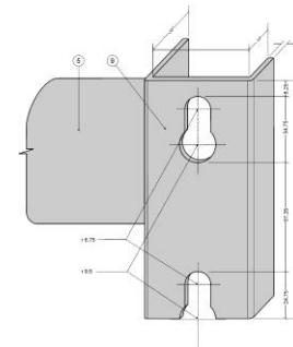
Fig. 10 – Sistema de encaixe Longarinas escala 1:1 (em mm)
