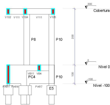
Corte D-D escala 1:50
