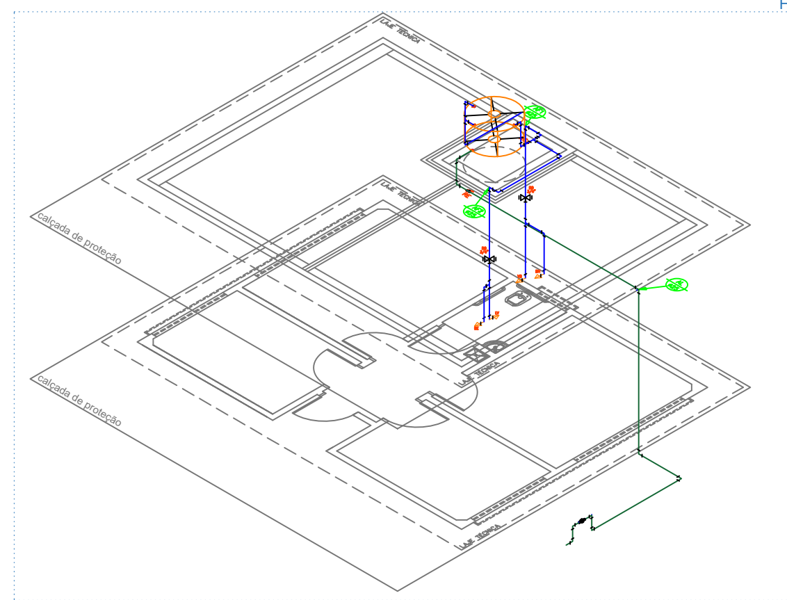
Detalhe Hidráulico Alimentação Escala 1:50
