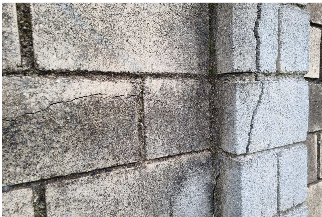
Trincas no muro da ESPC/GO
