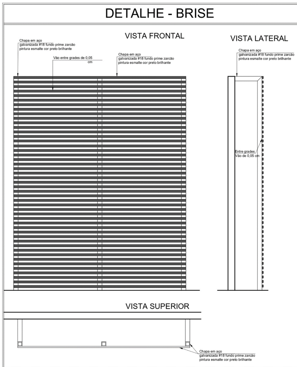
Figura 12 – Detalhamento de Brise
