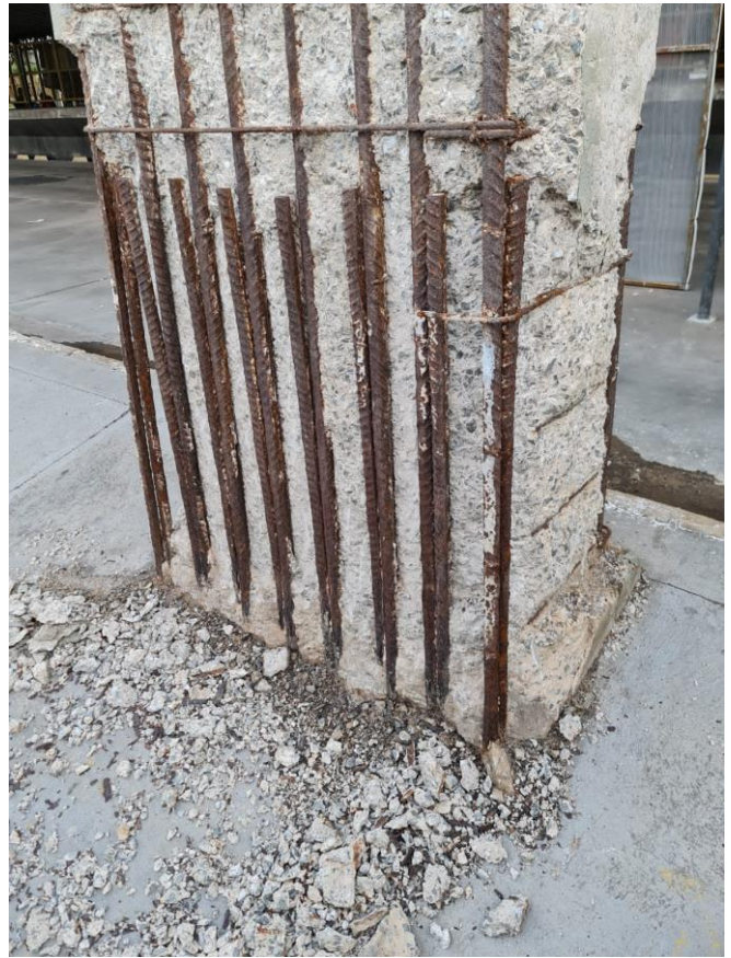
Amostra de pilar e viga com estrutura comprometida
