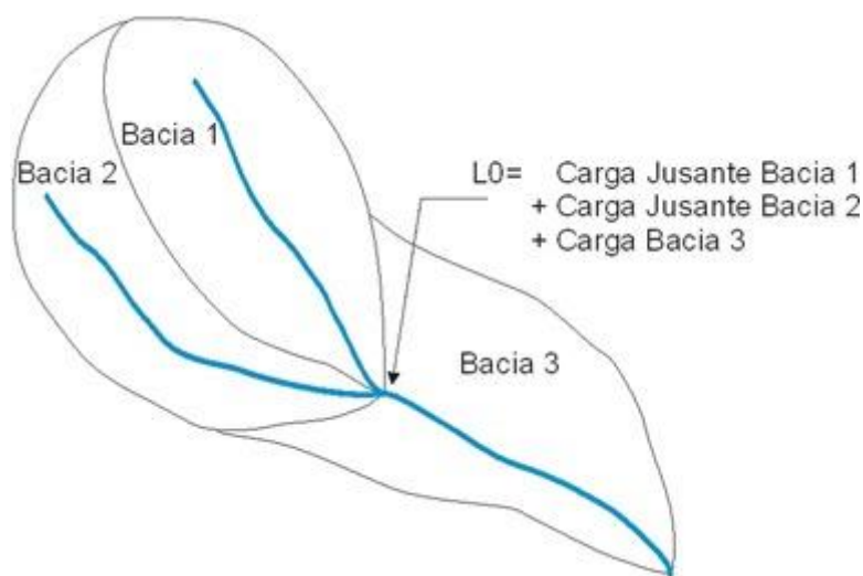
Figura 4 – Esquema de cálculo da carga inicial no trecho do modelo de qualidade da água.
