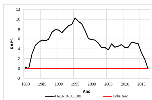
Figura 107 - Gráfico RAPS para vazão mínima de 90 dias da estação Fazenda Sucuri.
