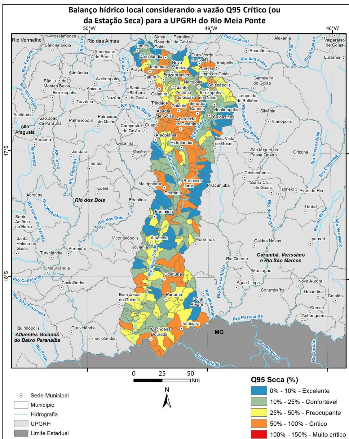
Figura 169 – Balanco hídrico local considerando a vazão Q95 Crítico (ou da Estação Seca) para a da UPGRH do Rio Meia Ponte.
