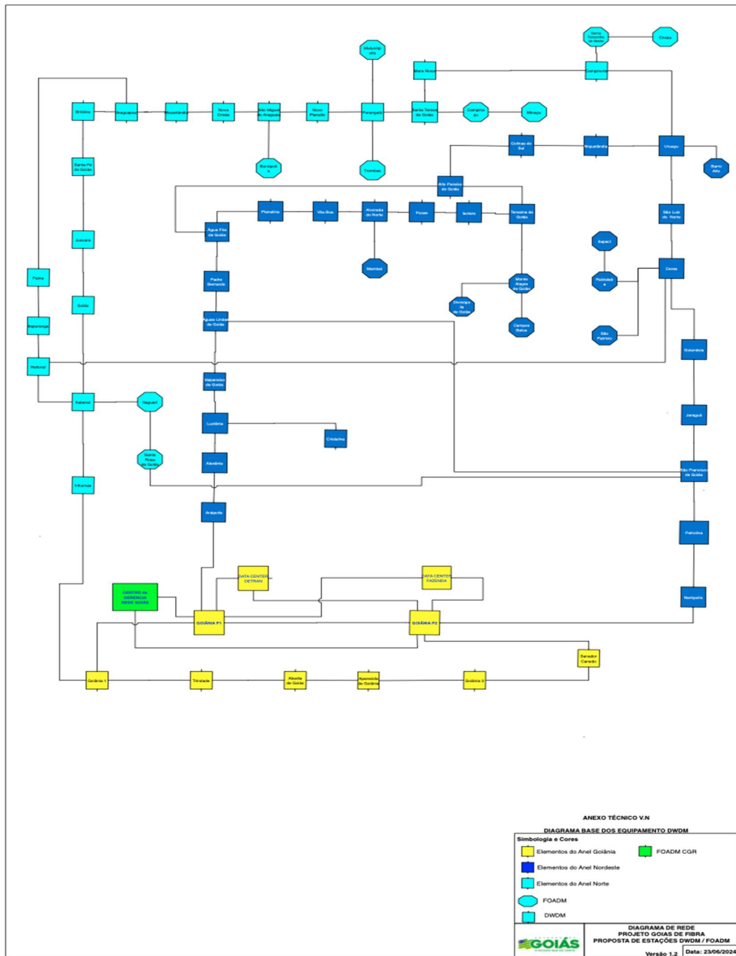
Figura 21: Rede DWDM do Anexo
