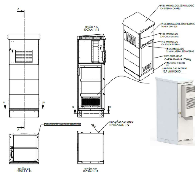
Figura 15: Modelos de Gabinete outdoor com sistemas de climatização 10.000BTU
