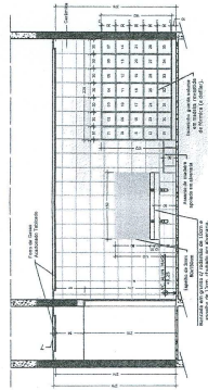
CORTE "B-B"
