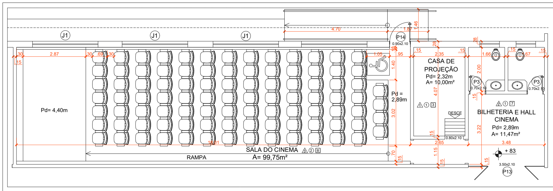
PLANTA BAIXA - CINE CULTURA
