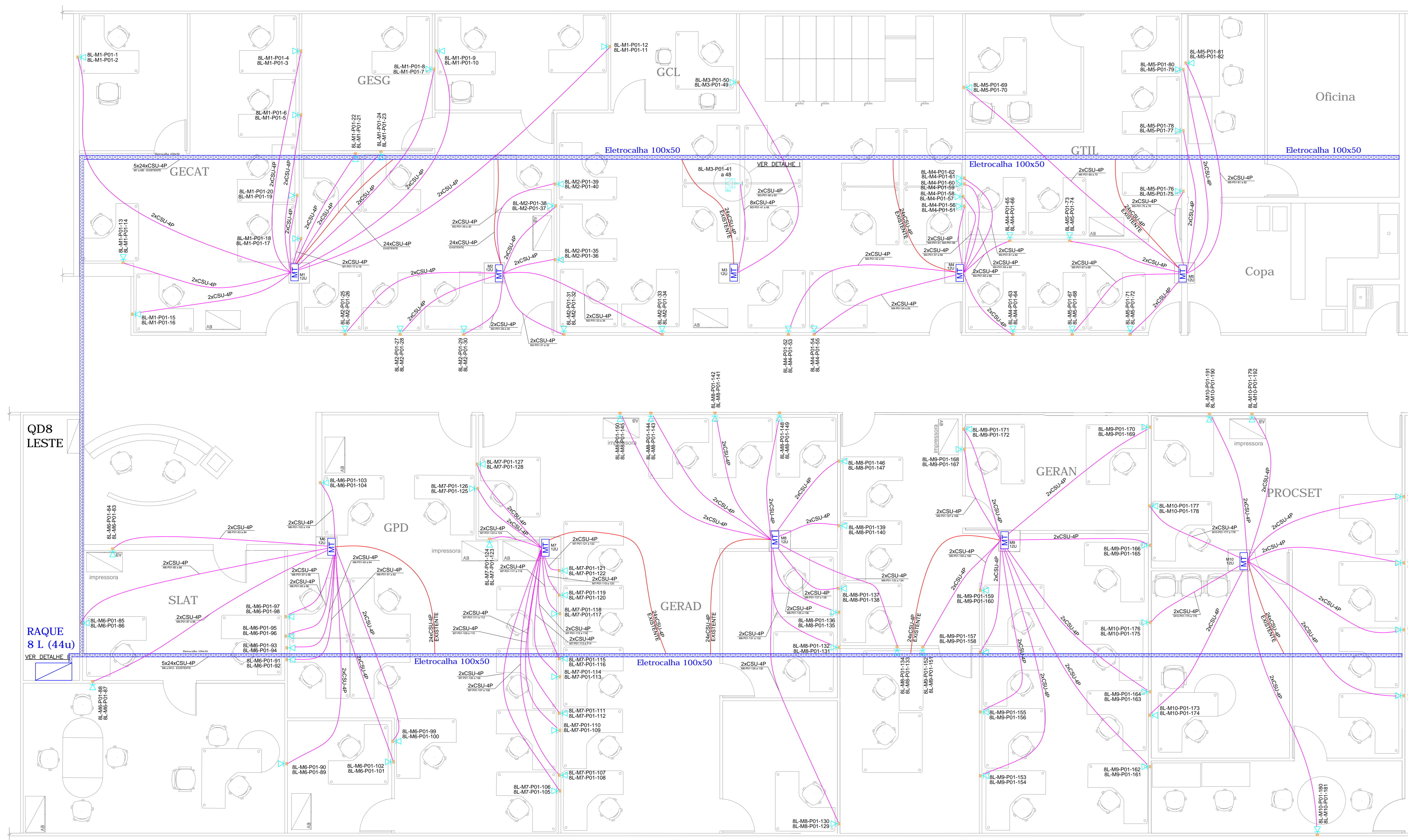
CABEAMENTO ESTRUTURADO – PLANTA BAIXA ESCALA: 1/50
