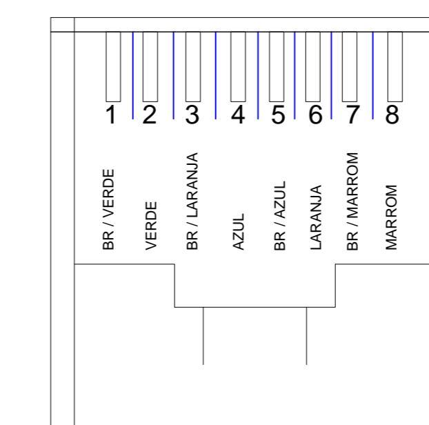
DETALHE DE TOMADAS RJ-45 CATEGORIA 5e – EIA/TIA – 568A MODULAR JACK 8 POSIÇÕES ESCALA: S/ESCALA
