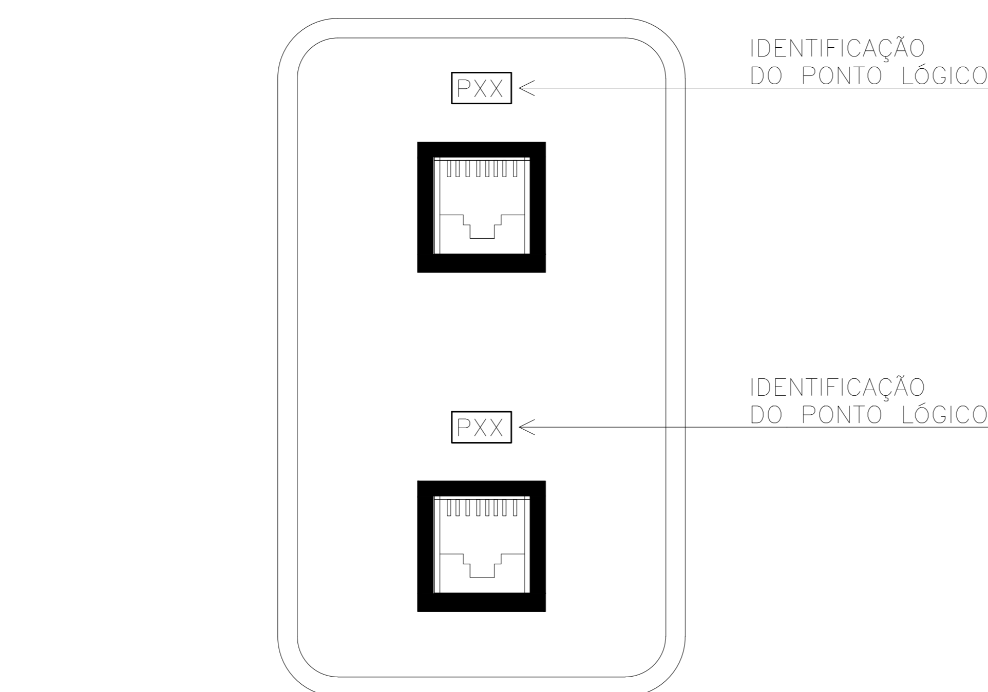
DETALHE DE TOMADAS DE DADOS (2 RJ-45) EM CAIXA 4X2” ESCALA: S/ESCALA
