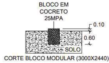
CORTE BLOCO MODULAR (3000X2440)
