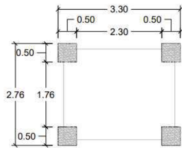
PLANTA BASE MODULAR (3000 X 2440)
