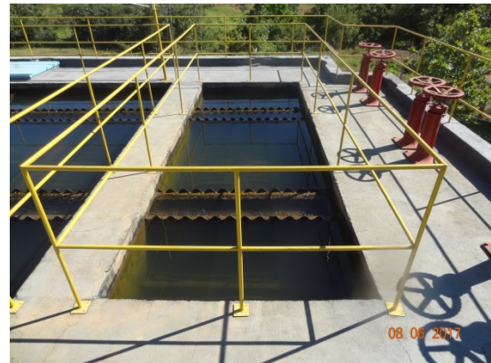
Foto 8 – ETA/ Floculadores com guarda-corpos recuperados e pintados
