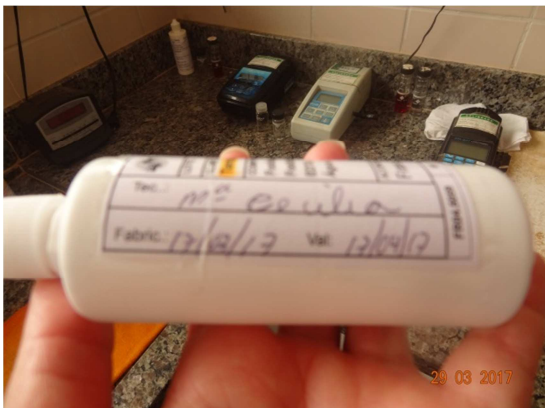
Foto 3 – Reagentes com datas atualizadas
