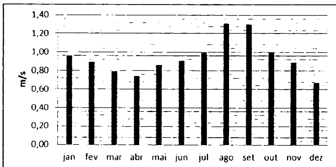
Figura 6. Gráfico da variação anual da velocidade dos ventos no período de 2003 a 2013.
