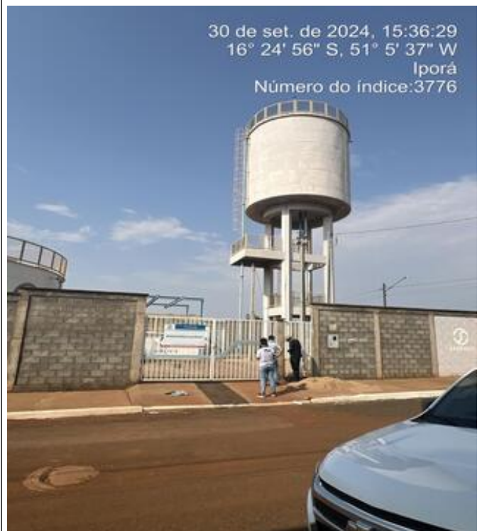
Foto 06 - REL/200 m 3 concreto instalado e operando.
