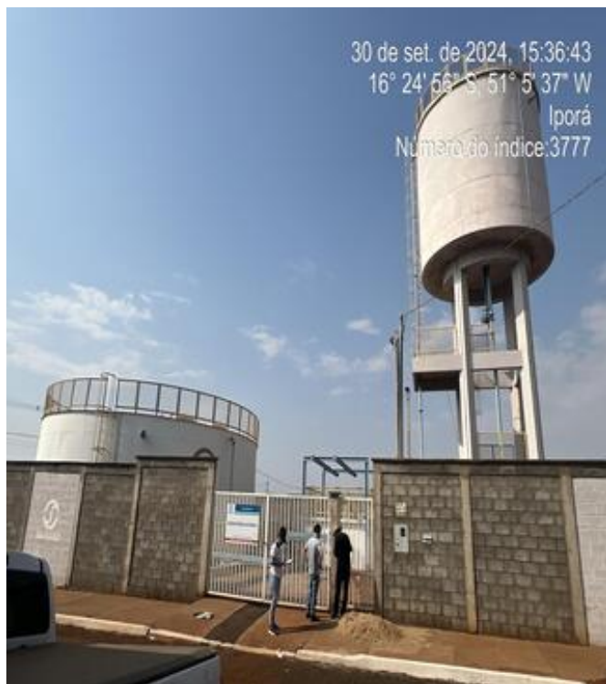
Foto 05 - RAP/500 m 3 metálico instalado e operando.
