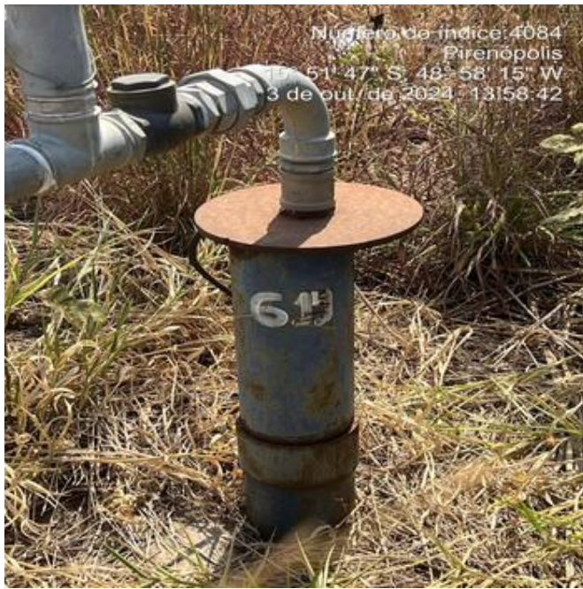
Foto 1 - Poço 614 interligado ao SAA, porém está aguardando instalação de filtro.
