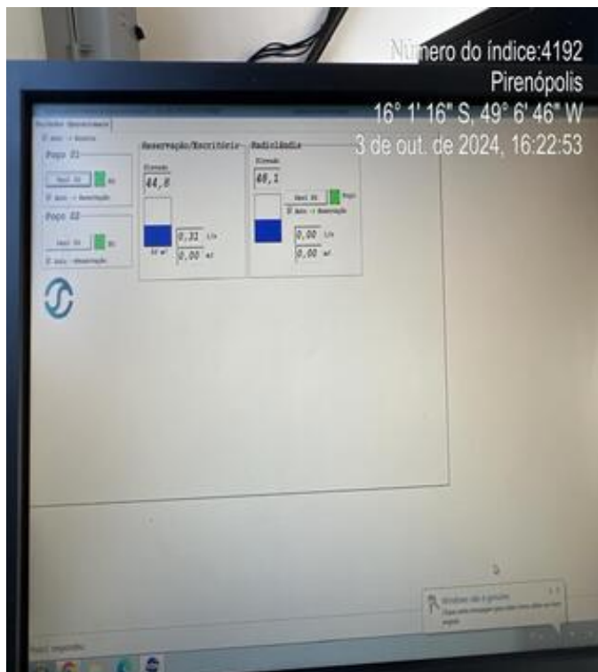
Foto 1 - Supervisório do subdistrito de Jaranápolis. REL/50 m 3 com 44,8% de reserva.
