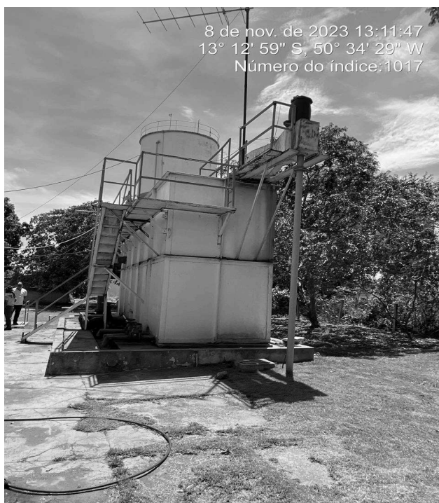
Foto 3 - ETA Compacta com pintura desgastada.
