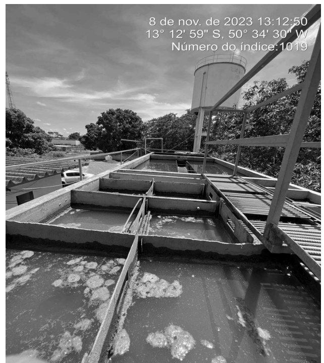
Foto 6 - ETA/Floculadores, Decantação e Filtração.
