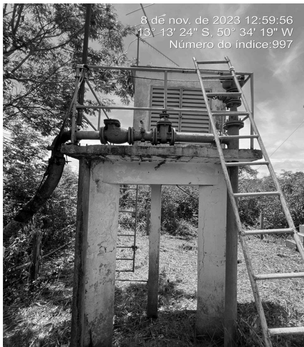
Foto 1 - Captação/EEAB com pintura desgastada e perda de revestimento e ferragem exposta.
