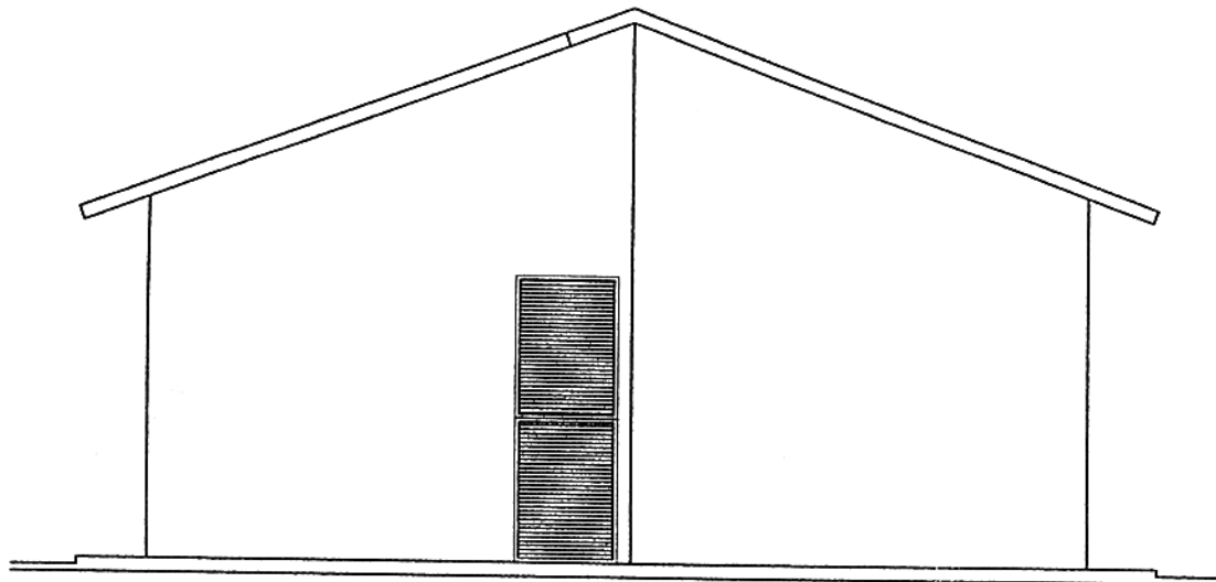
Fachada Posterior ESC.:1/50
