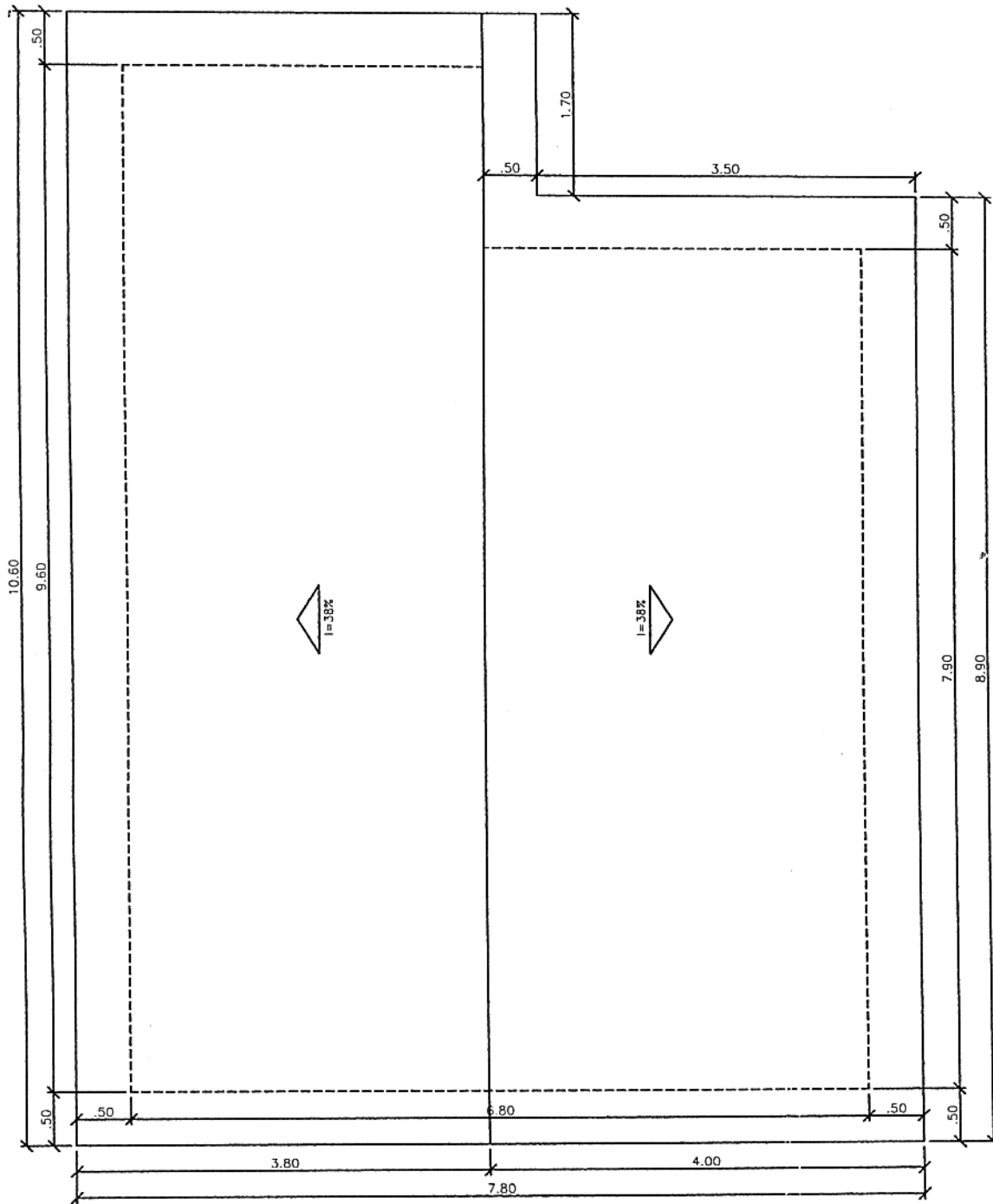
Cobertura ESC.:1/50
