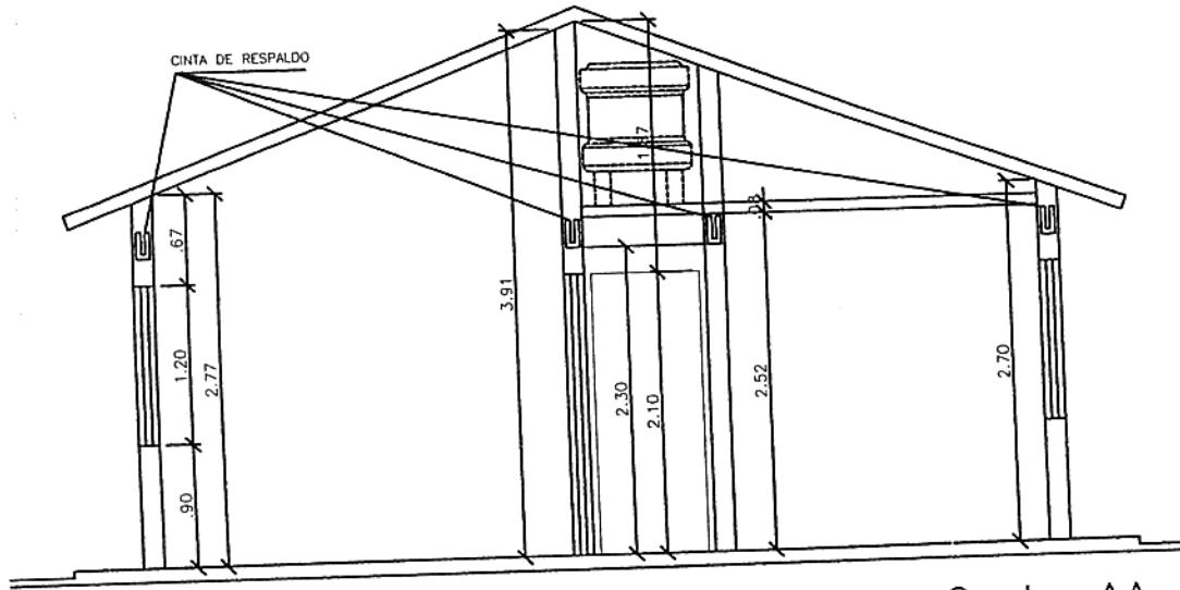
Corte AA ESC.:1/50
