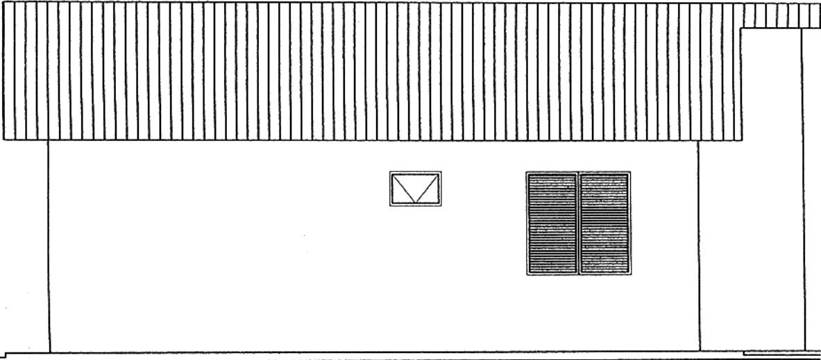
Fachada Lat. Direita SEM ESC.
