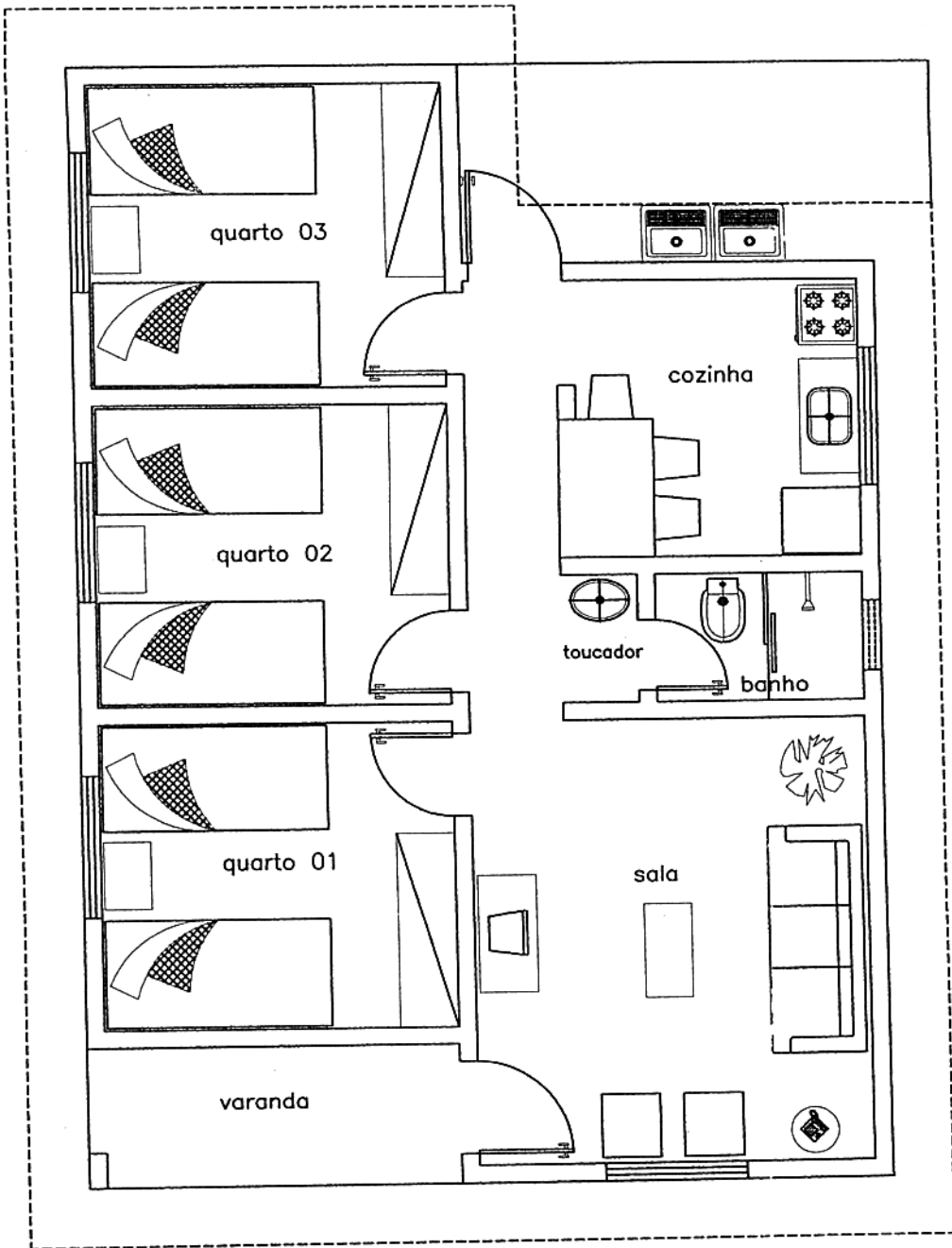
Layout ESC.:1/100
