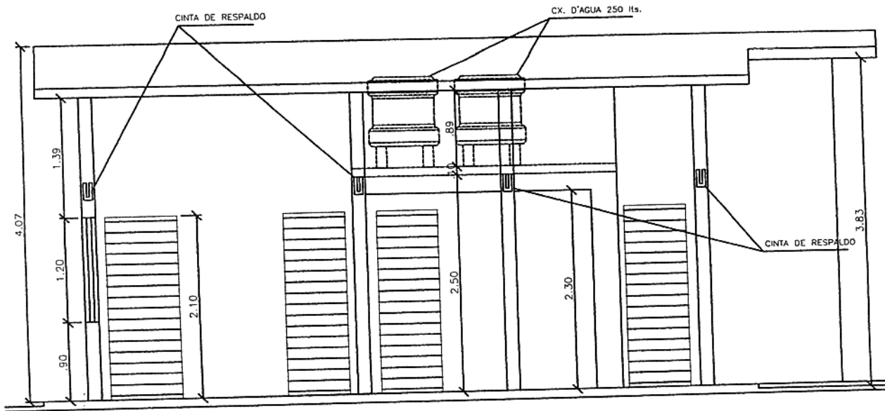
Corte BB SEM ESC.
