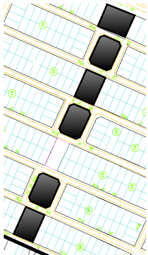
PROJETO URBANÍSTICO DETALHE 13 ESCALA 1:2.000
