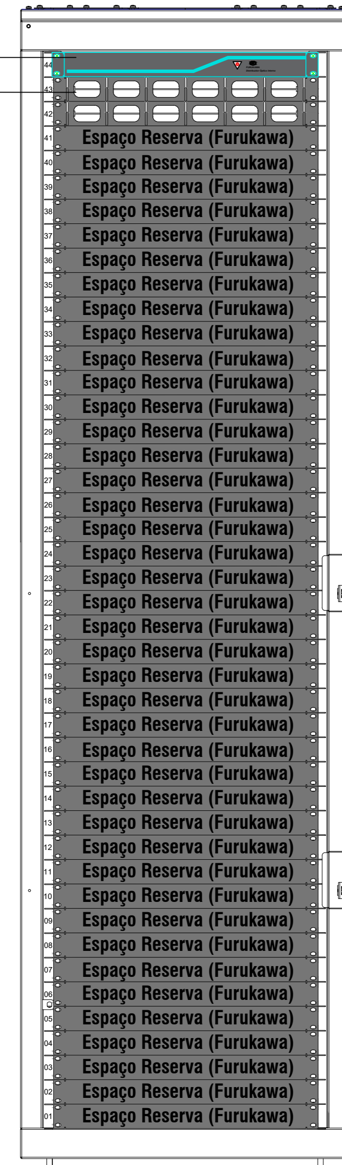
RACK FRONTA 44U - RACK 01 S/ESCALA
