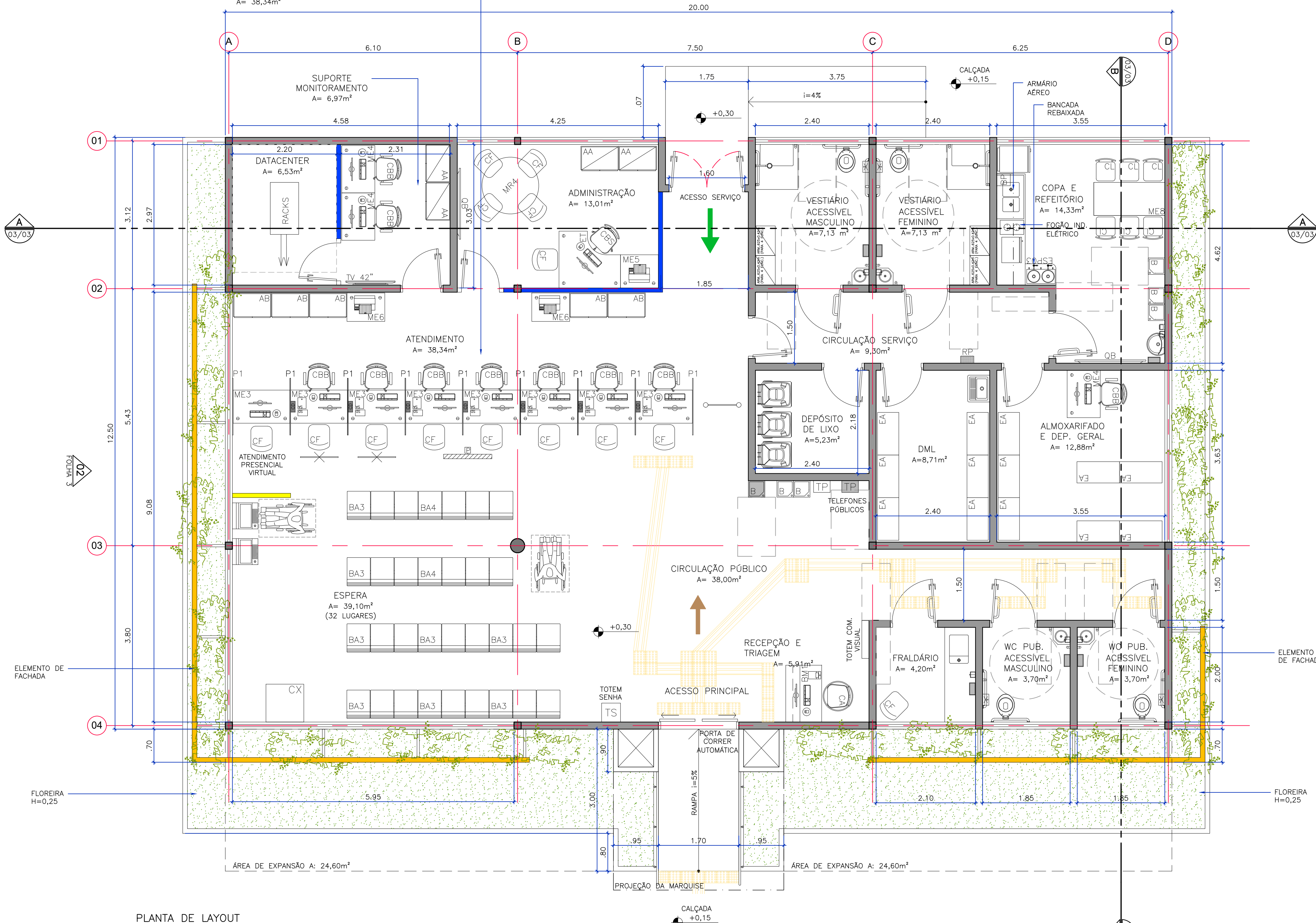
PLANTA DE LAYOUT ESCALA 1:50
